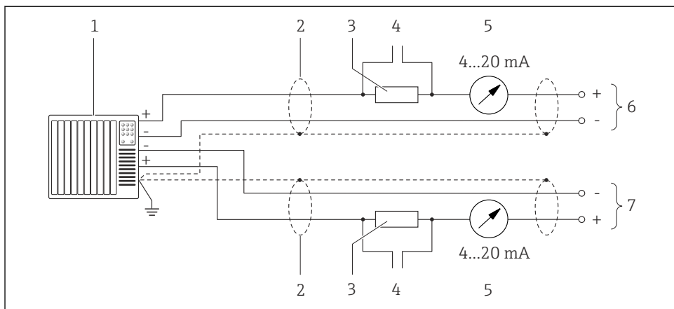
10 Exemplo de conexão para entrada HART (modo mestre) através da saída de corrente (ativa)
