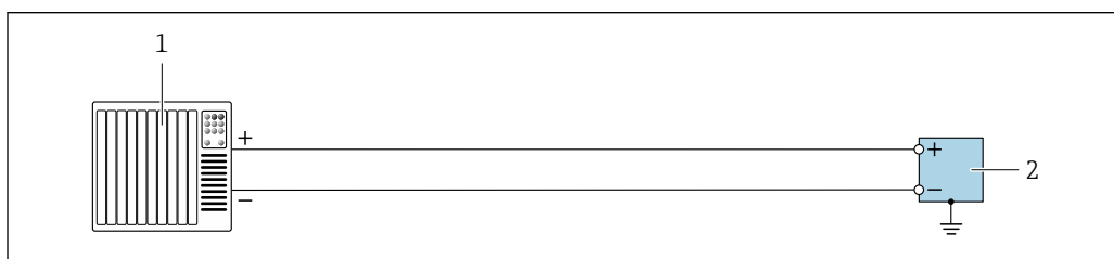
12 Exemple de raccordement pour sortie impulsion / sortie fréquence / sortie tout ou rien (active)
