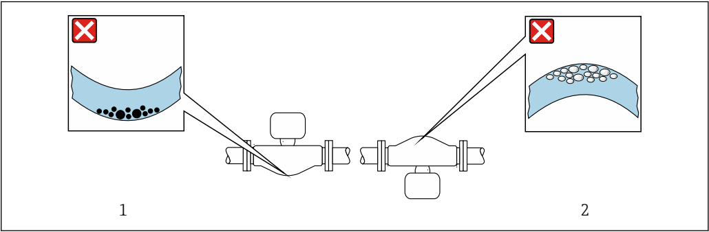
14 弓形計測チューブセンサの取付方向
