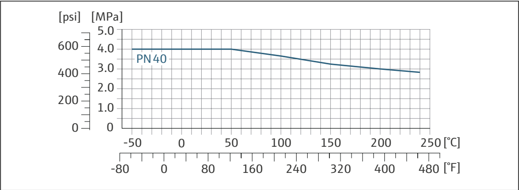
図 21 フランジ材質 1.4301 (SUS F304 相当) ; 接液部 アロイ C22
