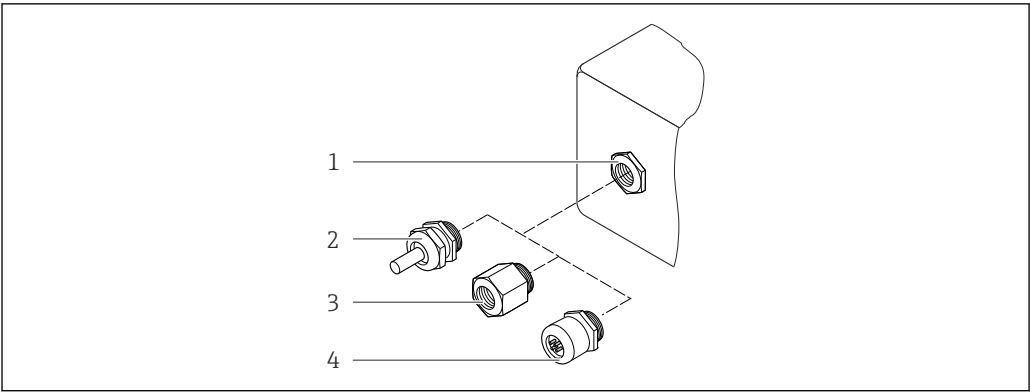
図 40 可能な電線口/ケーブルグランド
