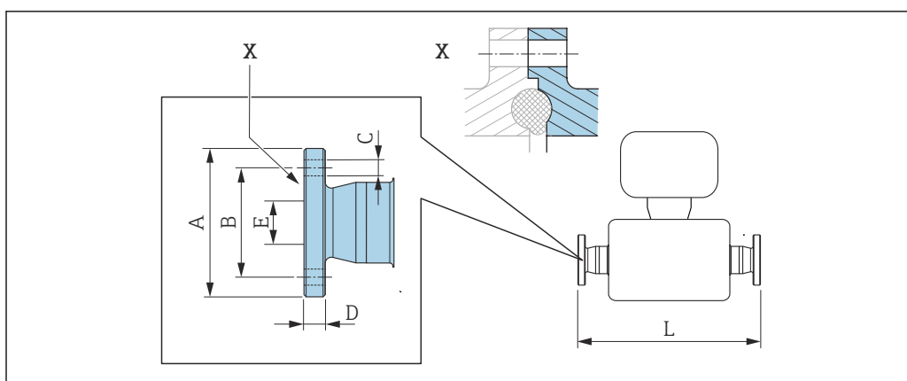
図 30 X の詳細：非対称型プロセス接続；着色部分が供給されます。
