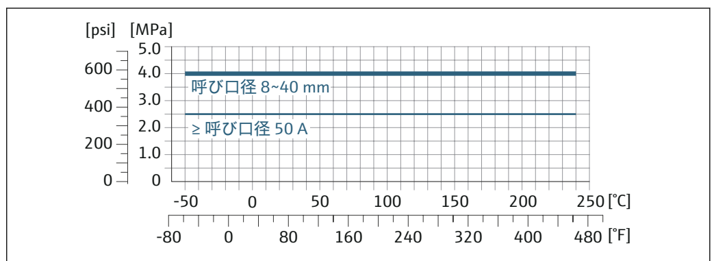
図 25 接続部の材質 1.4404 (SUS 316 相当または SUS 316L 相当)
