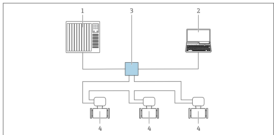
図 54 PROFINET ネットワーク経由のリモート操作オプション：リング型トポロジー
