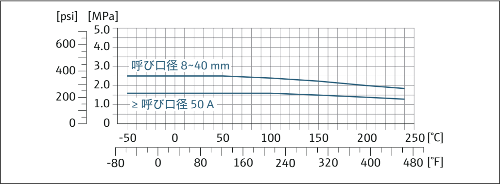
図 20 接続部の材質 1.4404 (SUS 316 相当または SUS 316L 相当)
