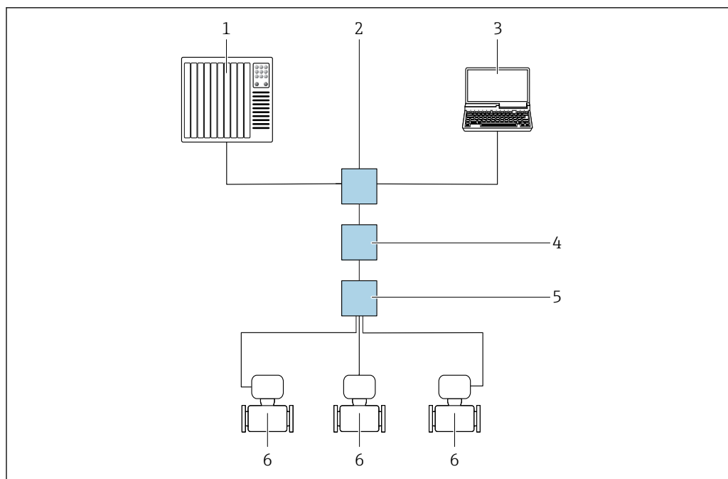
図 49 Modbus TCP over Ethernet-APL プロトコル経由のリモート操作用オプション（アクティブ）
