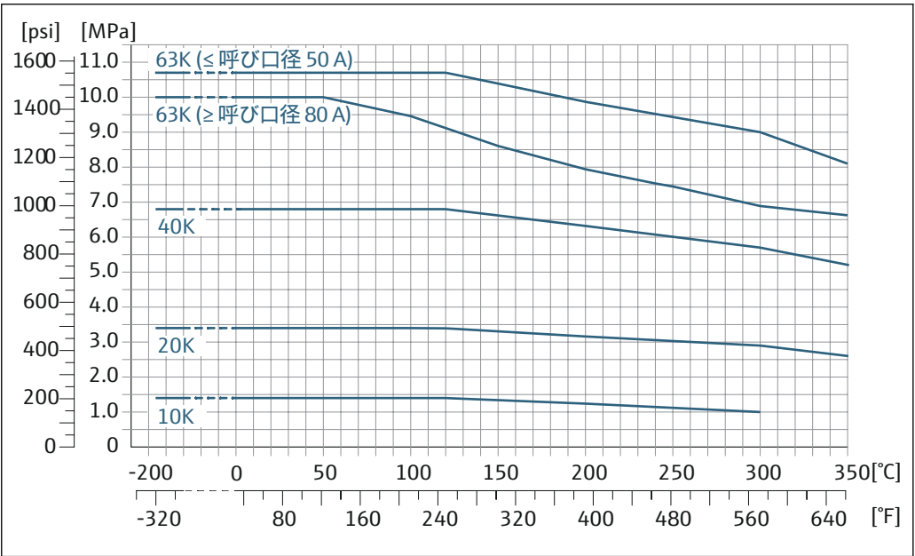
19 フランジ材質 1.4404 (SUS F316 相当または SUS F316L 相当)、アロイ C22
