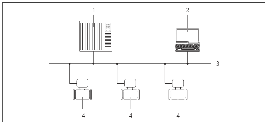
図 46 PROFIBUS DP ネットワークを介したリモート操作のオプション
