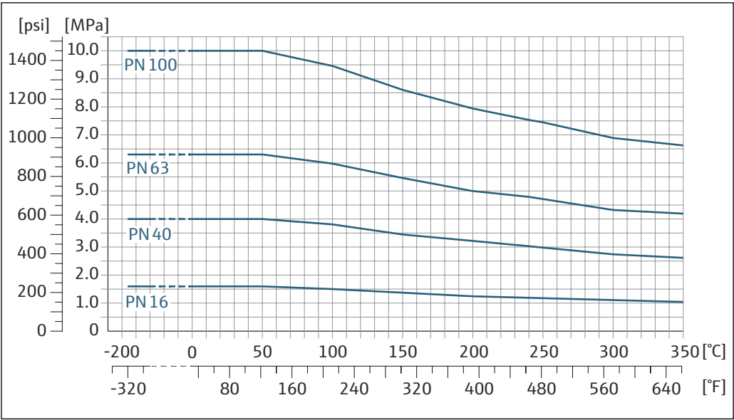
図 16 フランジ材質 1.4404 (SUS F316 相当または SUS F316L 相当)、アロイ C22
