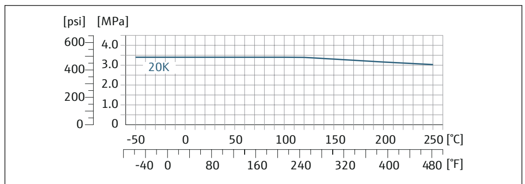
図 23 フランジ材質 1.4301 (SUS F304 相当) ; 接液部 アロイ C22
