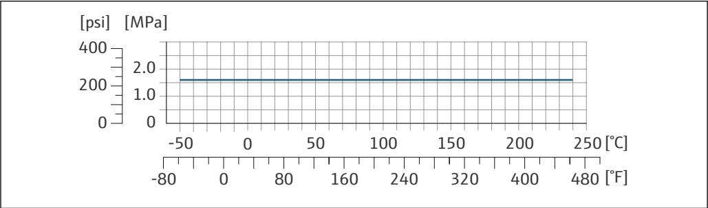
図 27 接続部の材質 1.4404 (SUS 316 相当または SUS 316L 相当)
