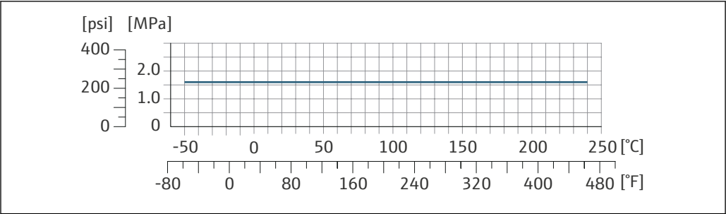
図 26 接続部の材質 1.4404 (SUS 316 相当または SUS 316L 相当)
