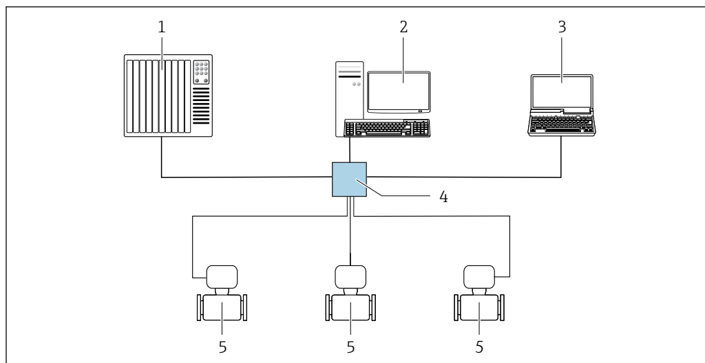
図 50 Modbus TCP over Ethernet - 100 Mbit/s 経由のリモート操作用オプション：スター型トポロジー
