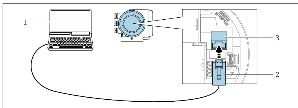
図 55 サービスインタフェース (CDI-RJ45) 経由の接続
