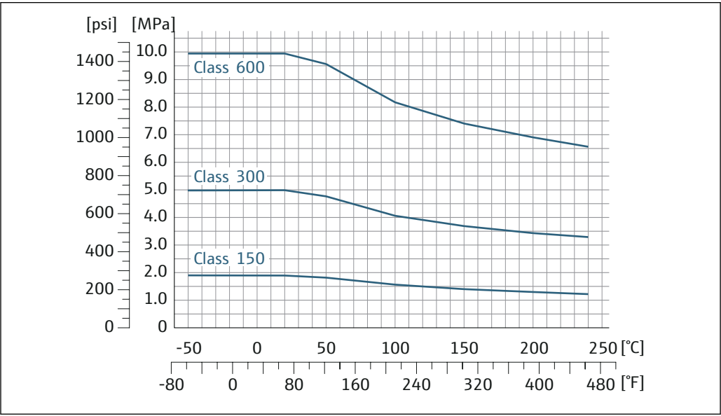
図 22 フランジ材質 1.4301 (SUS F304 相当) ; 接液部 アロイ C22
