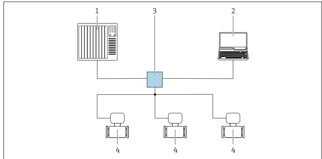
図 53 PROFINET ネットワーク経由のリモート操作オプション：スター型トポロジー
