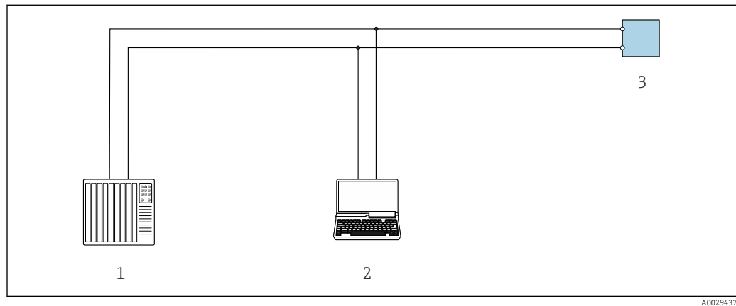
24 Möglichkeiten der Fernbedienung via Modbus-RS485-Protokoll (aktiv)
