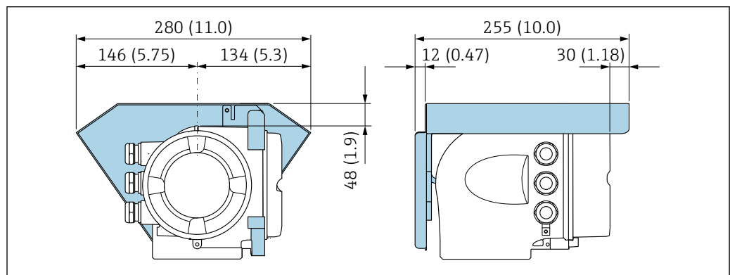
10 Tampa de proteção para Proline 500; unidade mm (pol.)
