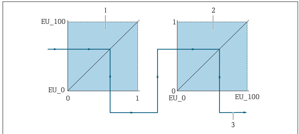
16 Scalatura del valore misurato nel Blocco Ingresso Analogico
