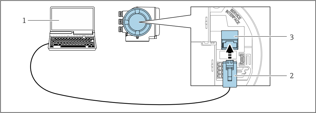
■ 26 サービスインタフェース (CDI-RJ45) 経由の接続
