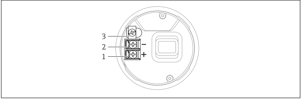
11 Bağlantı bölgesindeki bağlantı terminalleri ve toprak terminali, tek bölmeli muhafaza
