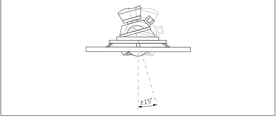
2 Hizalama ünitesine sahip anten gömme montaj
