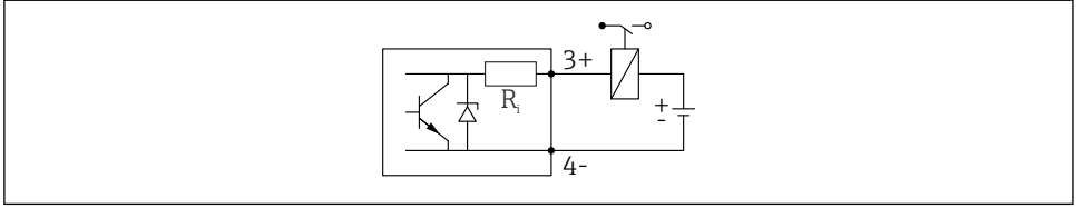
8 Röle bağlantısı örneği
