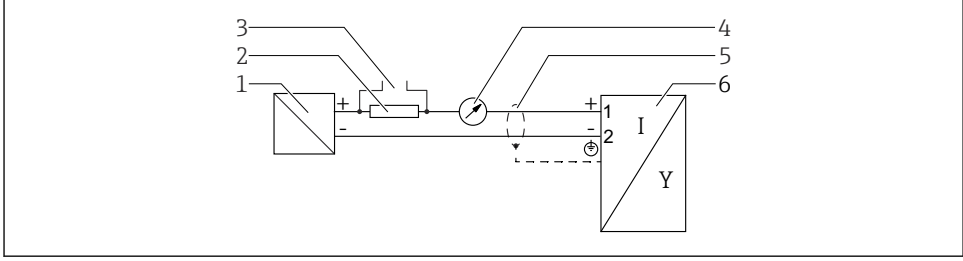
6 Fonksiyon şeması 4 ... 20 mA HART
