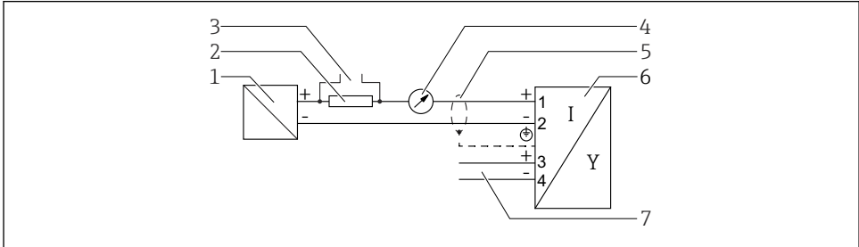
7 Fonksiyon şeması 4 ... 20 mA HART, anahtarlama çıkışı
