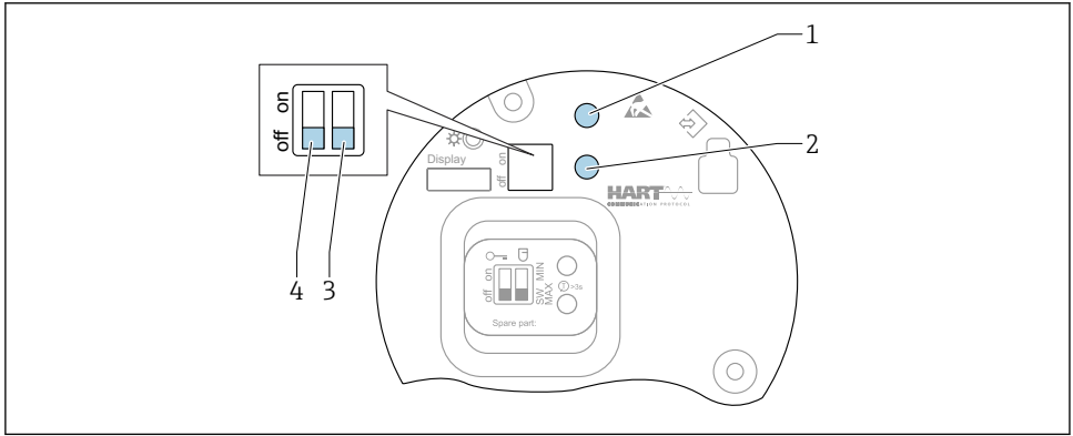
18 HART elektronik parçadaki çalıştırma tuşları ve DIP siviçler
