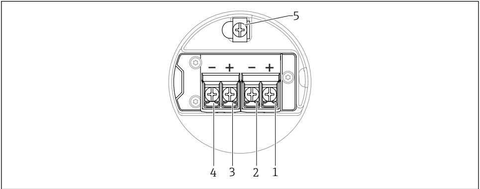
14 Bağlantı bölgesindeki terminal ataması; 4 ... 20 mA HART, anahtarlama çıkışı, çift bölmeli muhafaza
