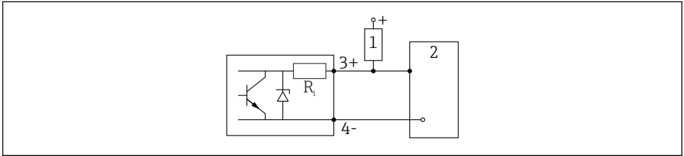
9 Dijital giriş için bağlantı örneği
