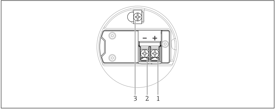
12 Bağlantı bölgesindeki terminal ataması; 4 ... 20 mA HART; çift bölmeli muhafaza
