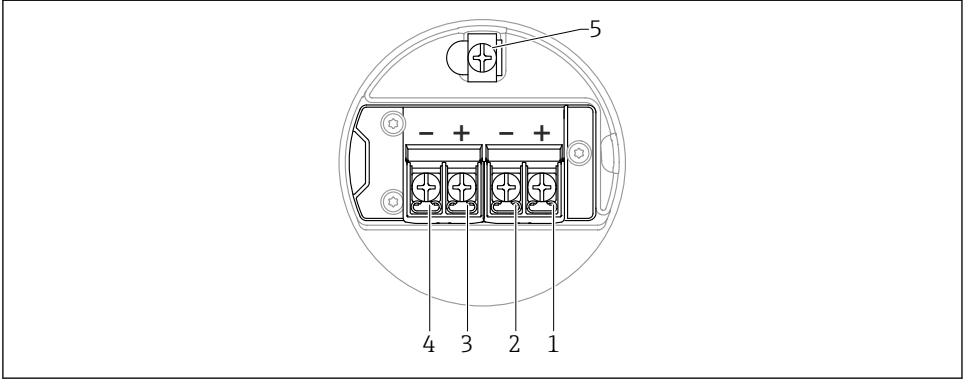
13 Bağlantı bölgesindeki terminal ataması; 4 ... 20 mA HART + 4 ... 20 mA analog; çift bölmeli muhafaza
