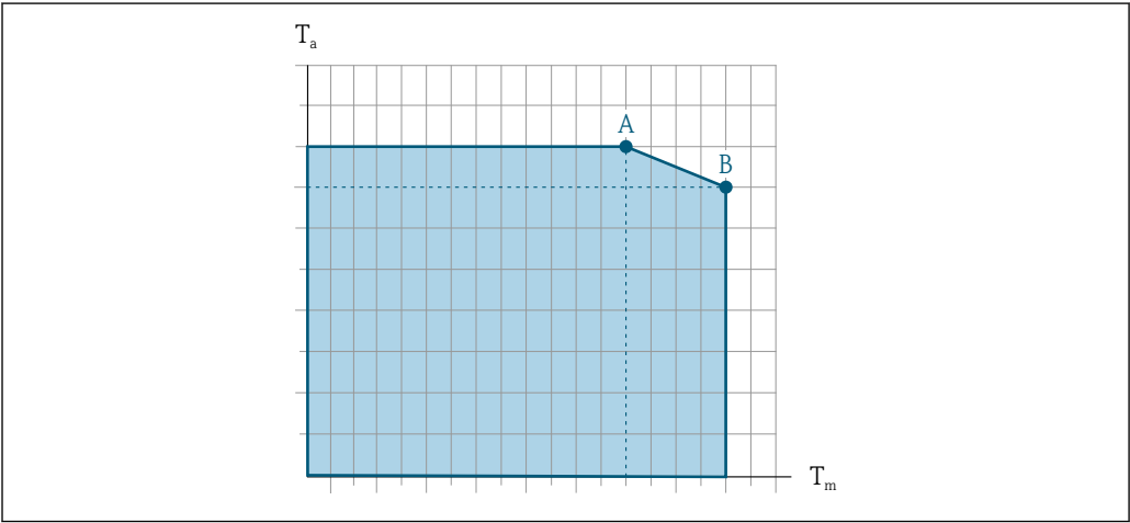
17 Representação exemplar, valores na tabela abaixo. T_a Temperatura ambiente T_m Temperatura do meio A Temperatura máxima permitida do meio T_m a T_{a\,máx.} = 60\,^{\circ}\text{C} (140 °F); temperaturas do meio mais altas T_m requerem uma redução na temperatura ambiente T_a B Temperatura ambiente T_a máxima permitida para a temperatura média T_m máxima especificada do sensor
