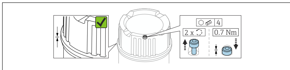
4 Cubierta con tornillo de fijación
