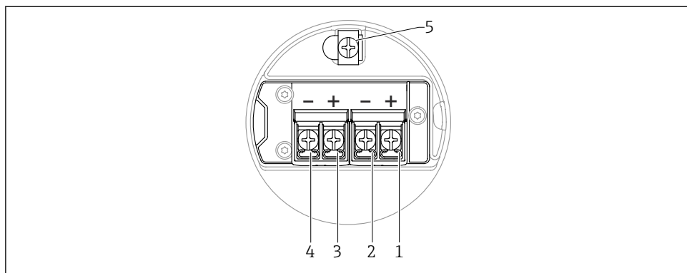
13 Asignación de terminales en el compartimento de conexiones; 4 ... 20 mA HART + 4 ... 20 mA analógico; caja de compartimento doble
