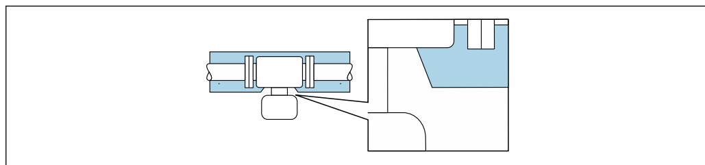
図 19 伸長ネックを覆わない断熱材：
