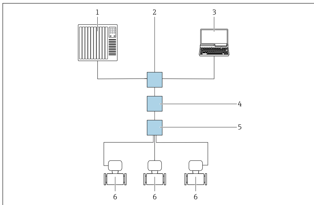
図 41 Modbus TCP over Ethernet-APL プロトコル経由のリモート操作用オプション（アクティブ）
