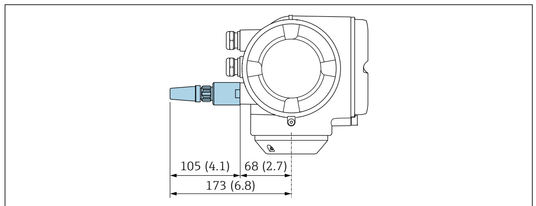
図 24 単位 mm (in)
