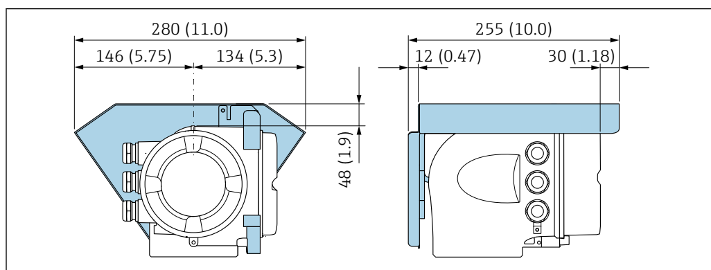
図 15 単位 mm (in)
