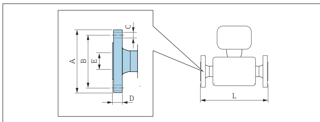
図 20 単位 mm (in)
