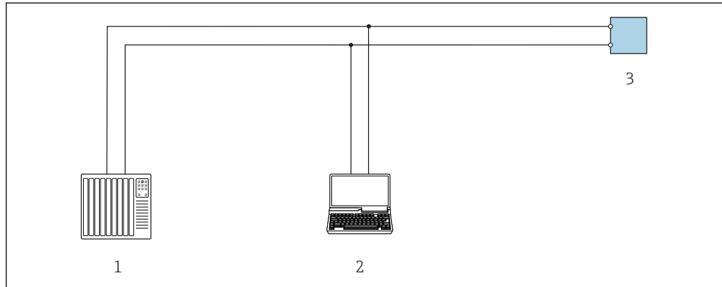
24 Möglichkeiten der Fernbedienung via Modbus-RS485-Protokoll (aktiv)
