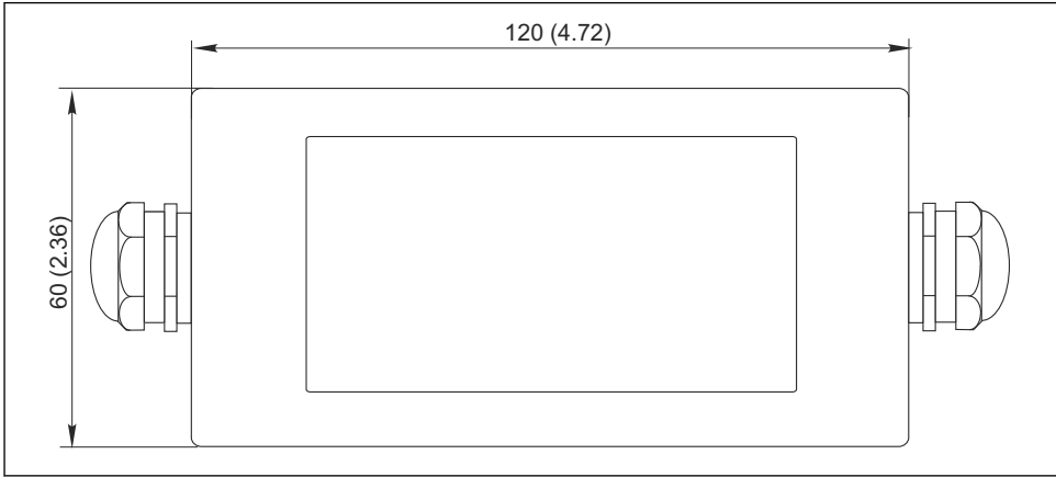
4 Üstten görünüm, boyutlar mm (inç) cinsindendir
