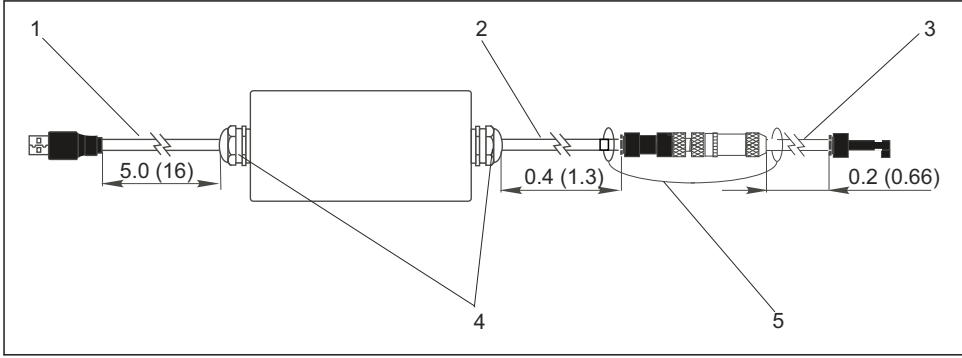
3 Commubox FXA291 ve bileşenleri, m (ft) cinsinden boyutlar
