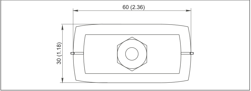
5 Yandan görünüm (CDI bağlantısı / cihaz tarafı), boyutlar mm (inç) cinsindendir
