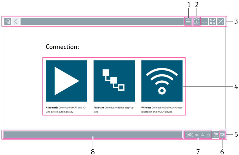
4 Exemple d'écran de démarrage
