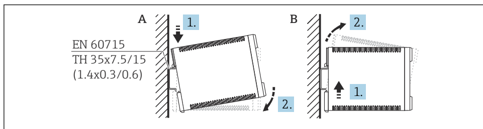
4 Montere/demontere DIN-skinnehuset. Måleenhet mm (in)
