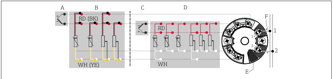
3 Asignación de las conexiones de terminales
