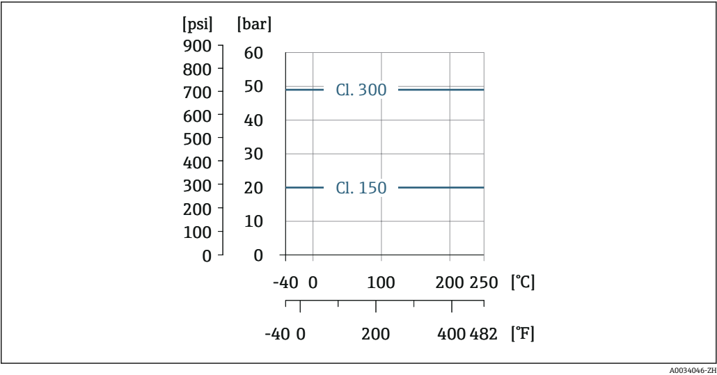
19 连接法兰的材质: 铸造合金 CX2MW, 类似 Alloy C22/2.4602 合金
