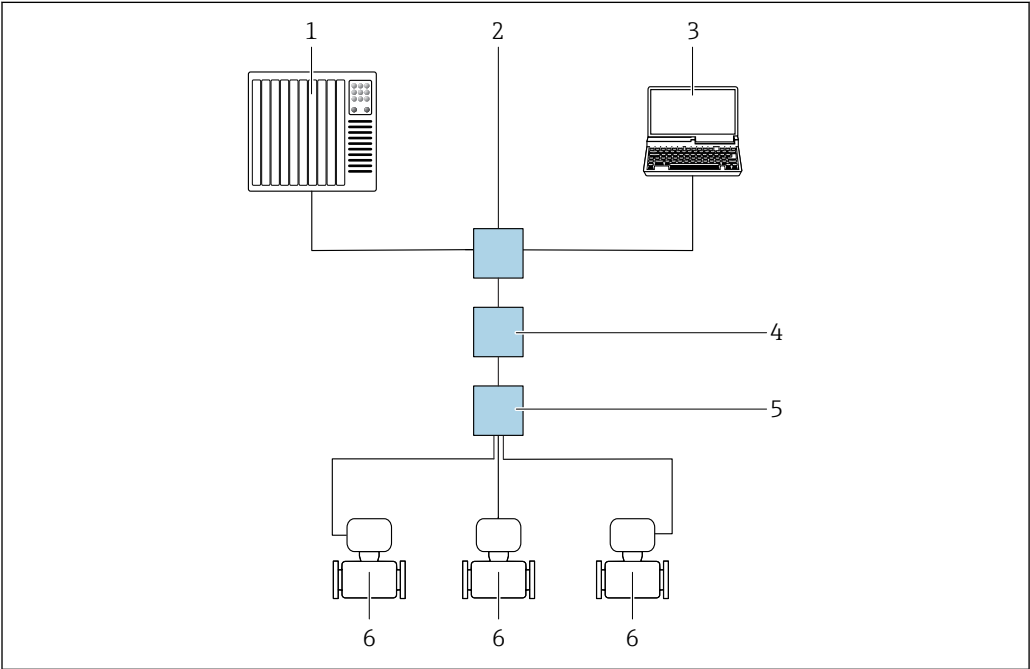
图 32 通过 Modbus TCP + Ethernet-APL 通信进行远程操作 (有源信号)
