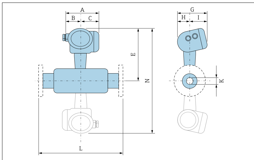
图 25 灰色区域：双传感器型
