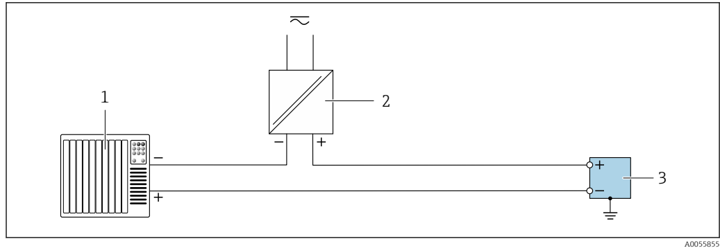
22 Exemple de raccordement pour sortie impulsion / sortie fréquence / sortie tout ou rien (passive)
