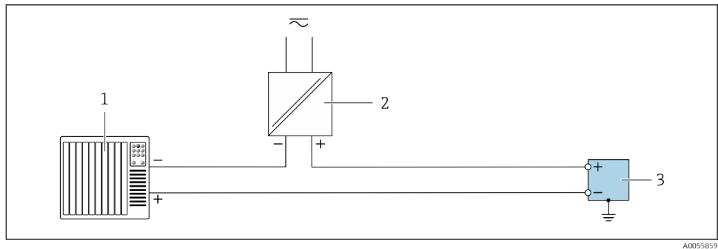
23 Exemple de raccordement pour sortie relais
