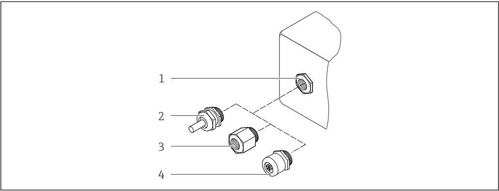
27 Possibilità di ingressi cavo/pressacavi
