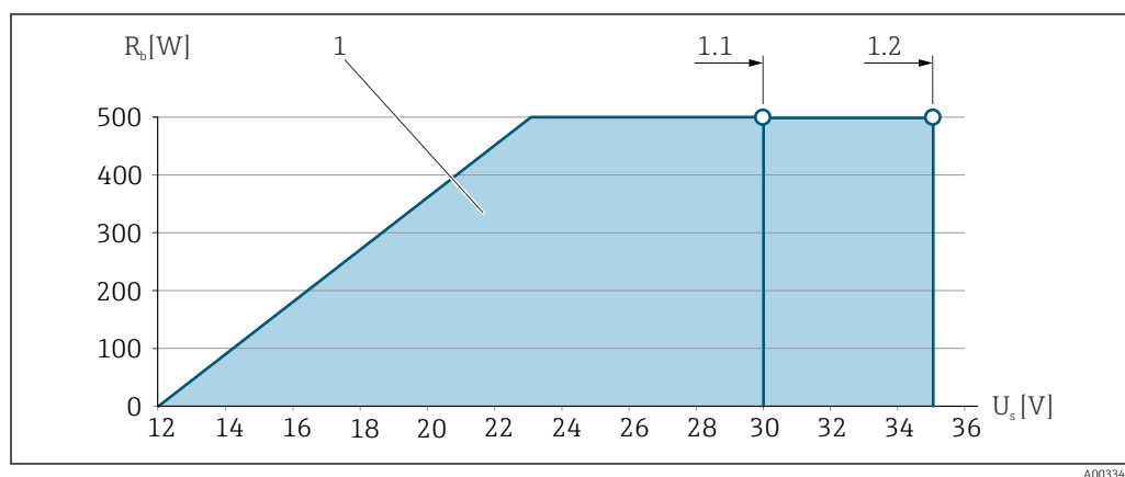
2 Carico per versione compatta senza display locale
