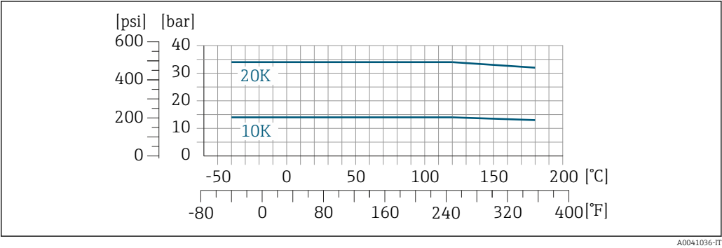
20 Materiale della connessione flangiata: acciaio inox, certificazioni multiple, 1.4404/F316/F316L
