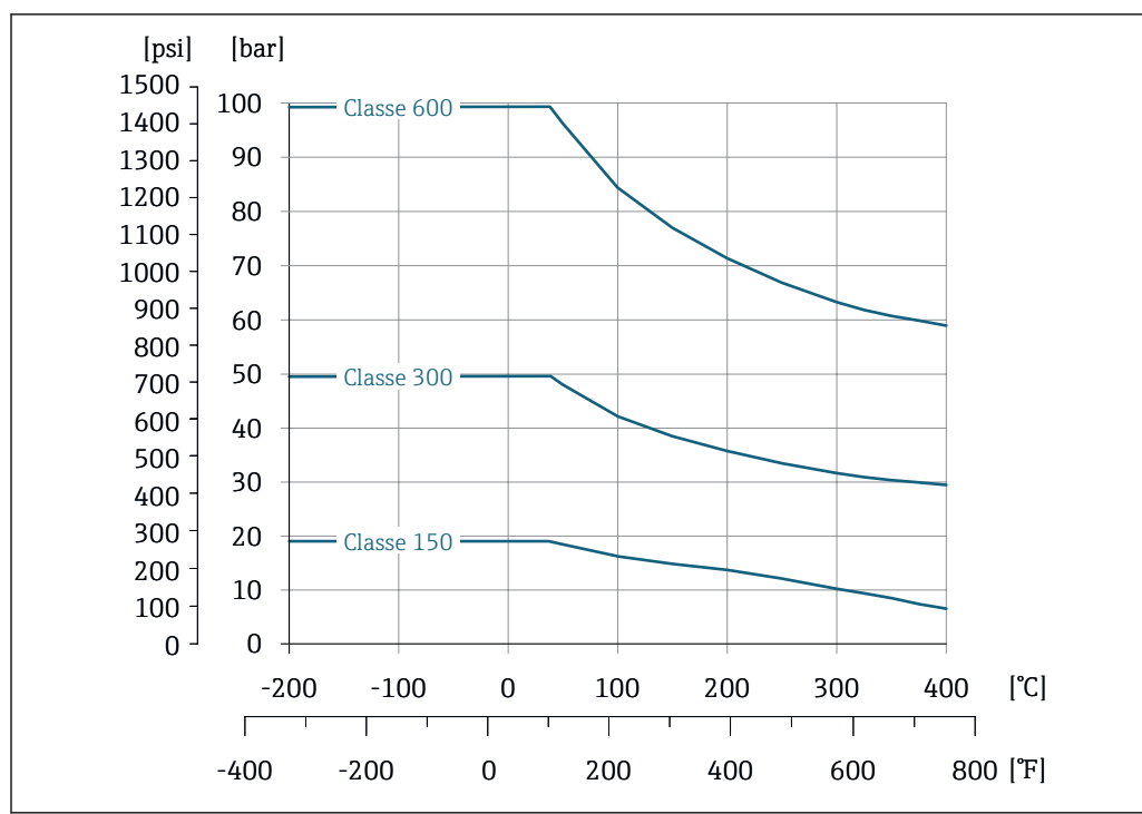
18 Materiale della connessione flangiata: acciaio inox, certificazioni multiple, 1.4404/F316/F316L
