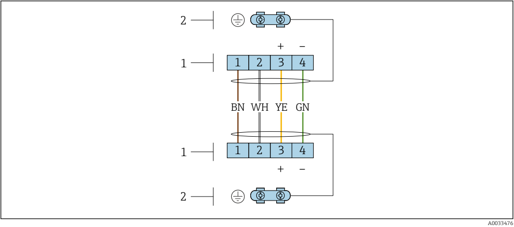
3 Morsetti per vano connessioni nel supporto da parete del trasmettitore e nella custodia di connessione del sensore 1 Morsetti per cavo di collegamento 2 Messa a terra mediante fermo serracavi
