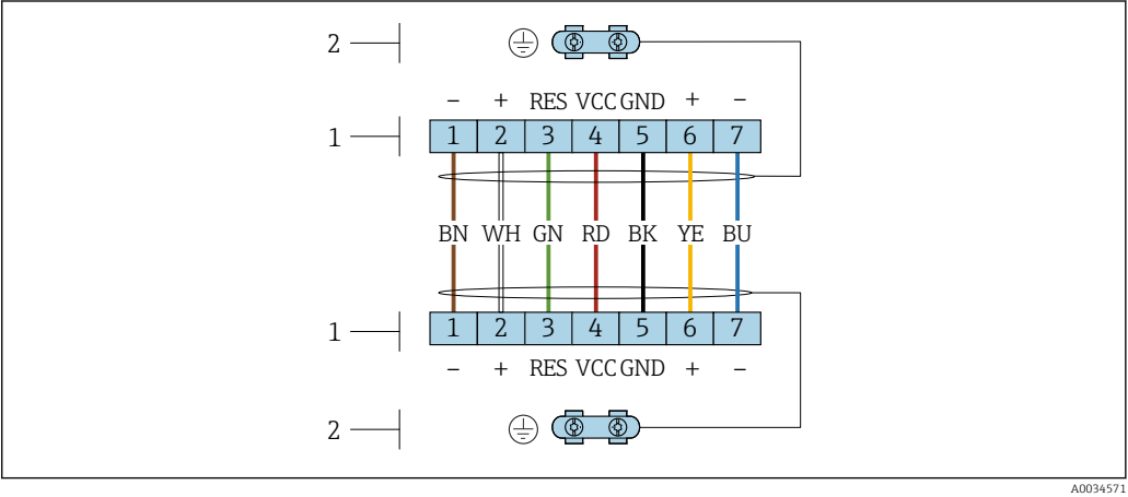
4 Morsetti per vano connessioni nel supporto da parete del trasmettitore e nella custodia di connessione del sensore 1 Morsetti per cavo di collegamento 2 Messa a terra mediante fermo serracavi
