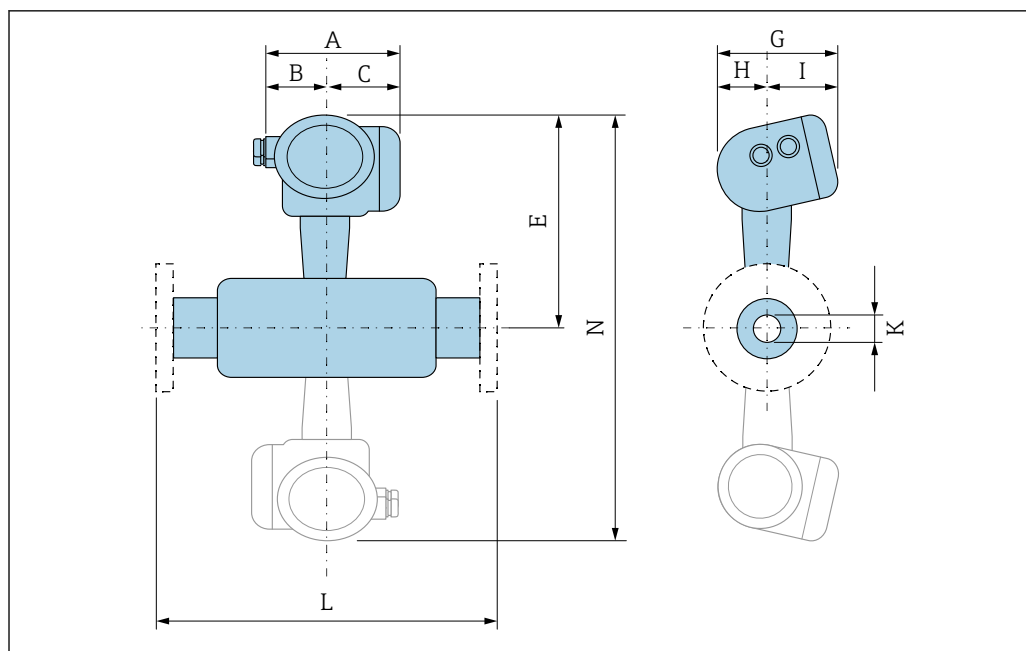
23 Parte ombreggiata: versione Dualsens
