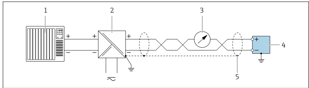
9 Esempio di collegamento all'uscita in corrente a 4 ... 20 mA con HART (passiva)
