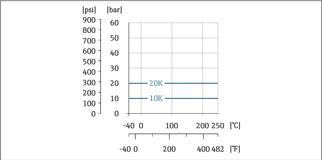
21 Materiale connessione flangiata: lega di fonderia, CX2MW simile ad Alloy C22/2.4602
