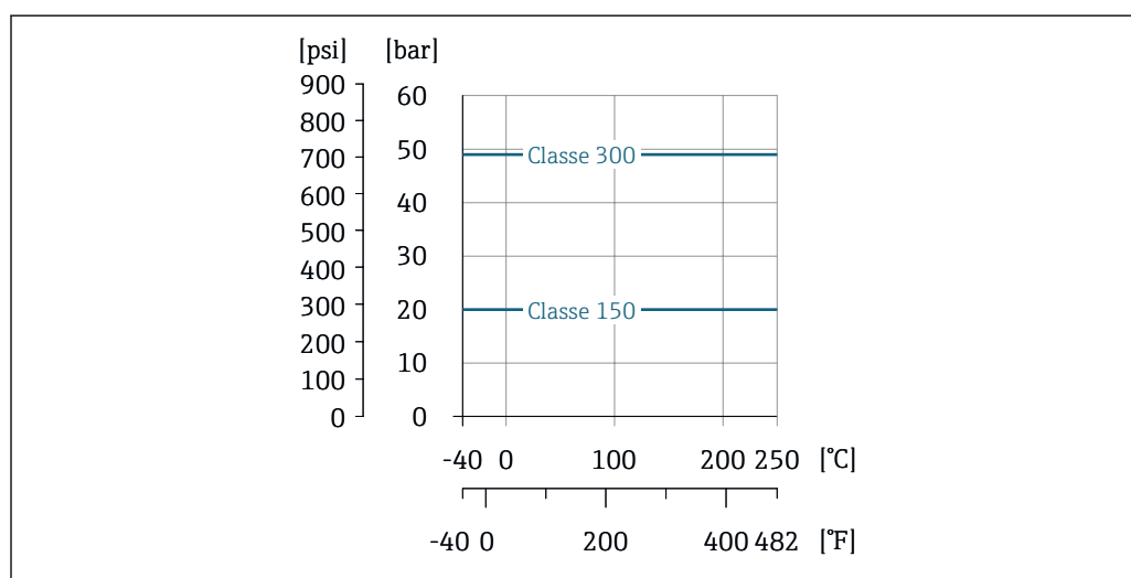
19 Materiale connessione flangiata: lega di fonderia, CX2MW simile ad Alloy C22/2.4602
