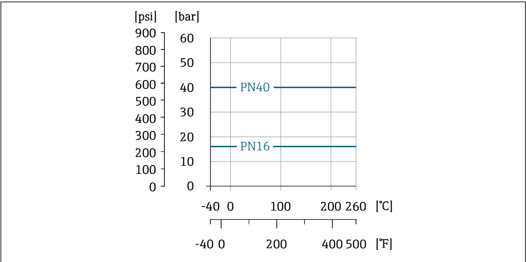
17 Materiale connessione flangiata: lega di fonderia, 2.4602/UNS N06022 simile ad Alloy C22/2.4602
