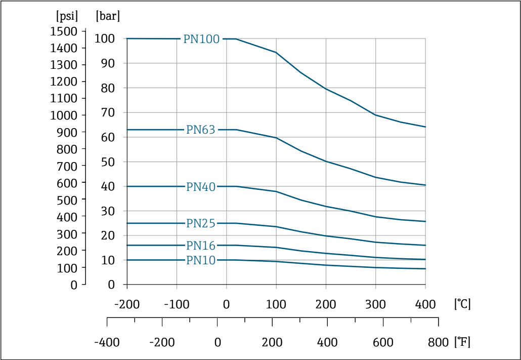
16 Materiale della connessione flangiata: acciaio inox, certificazioni multiple, 1.4404/F316/F316L
