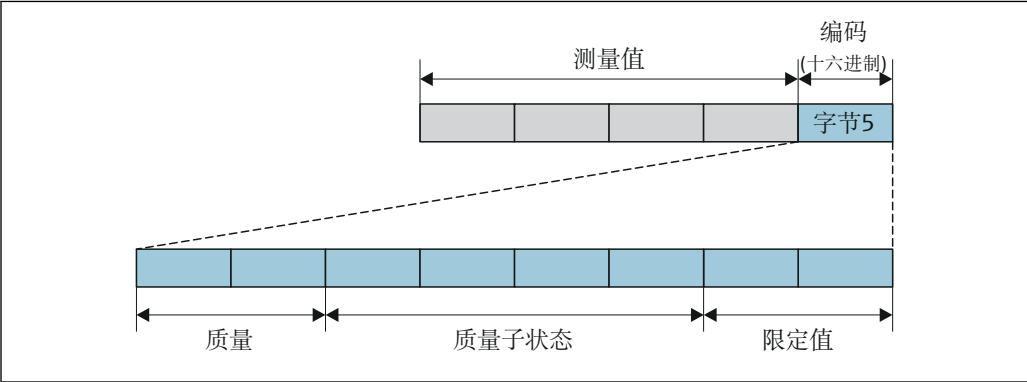
图 29 状态字节结构
