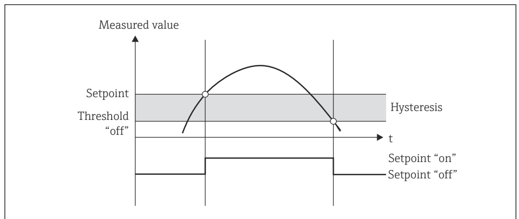
10 Рабочий режим MAX
