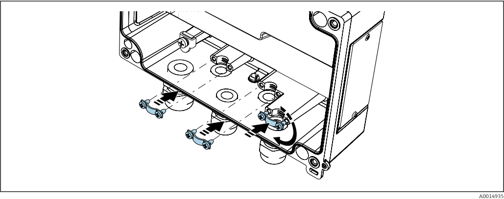
6 Соединение для заземления экрана
