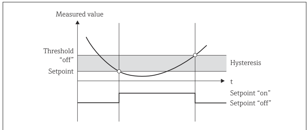
9 Рабочий режим MIN
