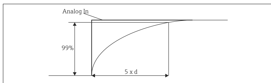
15 Демпфирование сигнала
