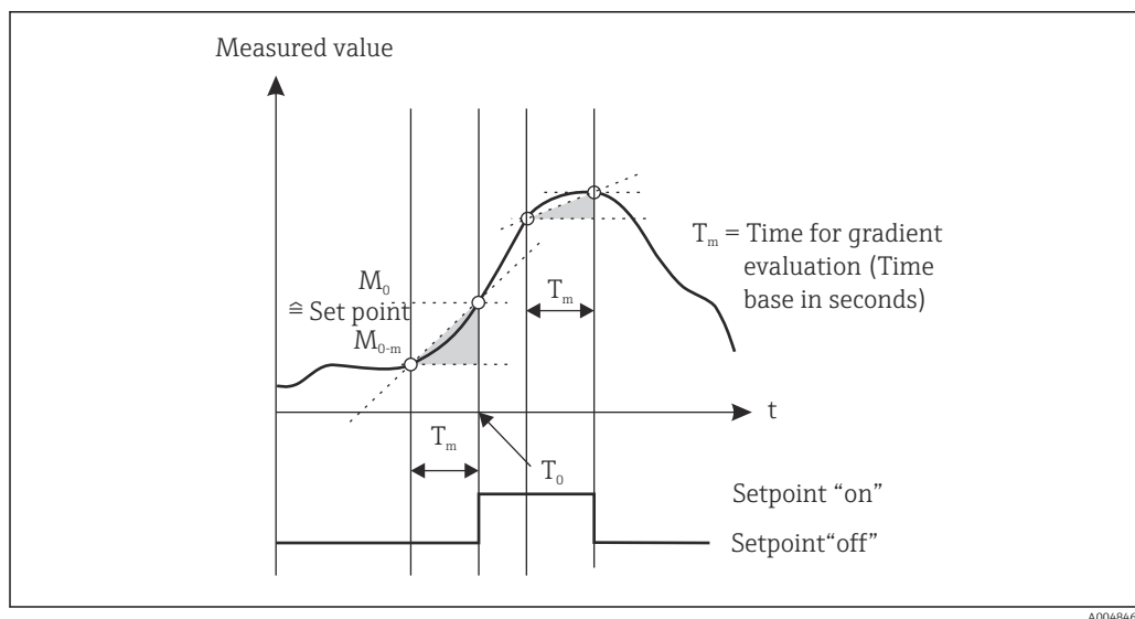
11 Режим работы Gradient (Градиент)
