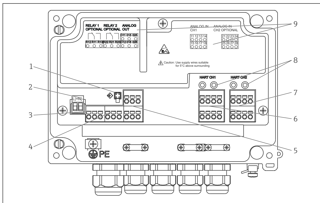
17 Вид изнутри и назначение клемм индикатора процесса
