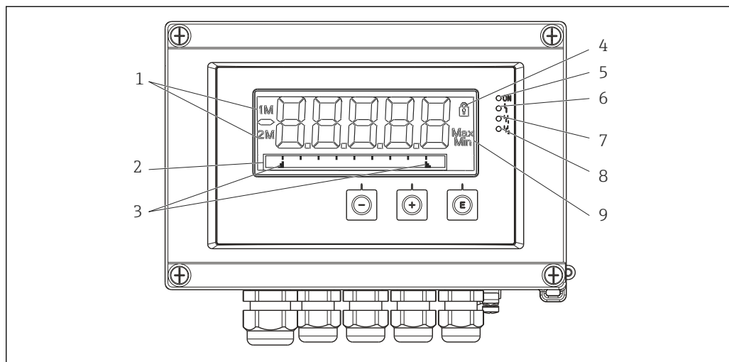
19 Дисплей индикатора процесса
