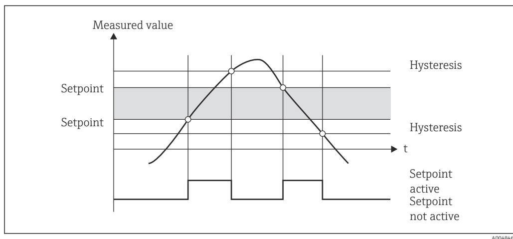
12 Режим работы OutBand (Внеполосный)
