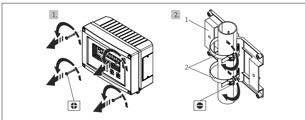
■ 2 Монтаж полевого индикатора на трубопроводе
