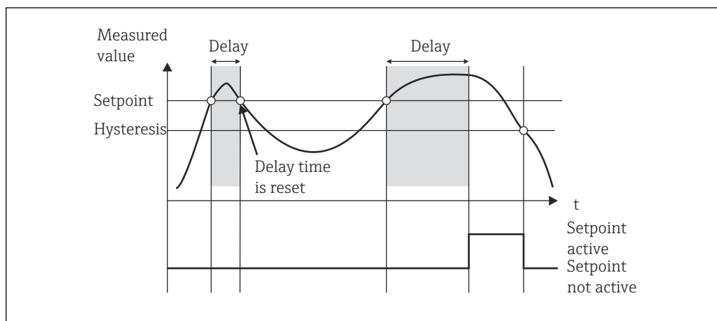
14 Активны и гистерезис, и задержка
