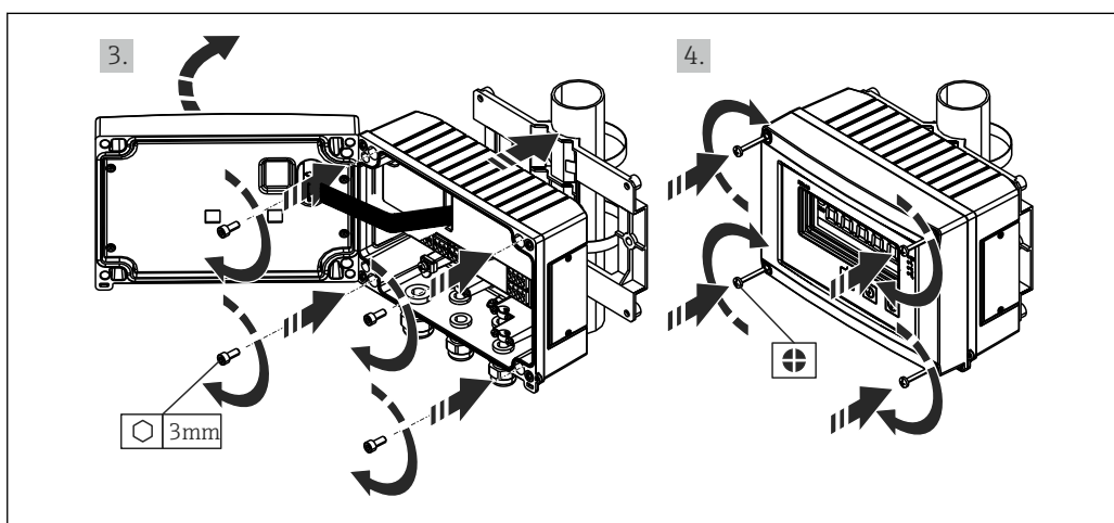
■ 3 Монтаж полевого индикатора на трубопроводе
