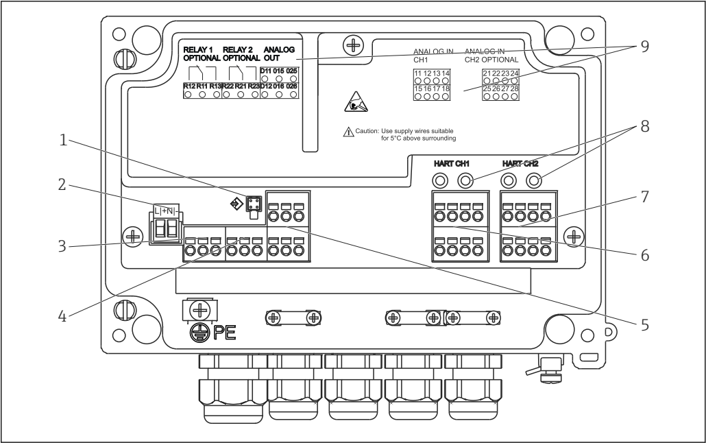
4 Назначение клемм прибора (канал 2 и реле являются опциональными компонентами)
