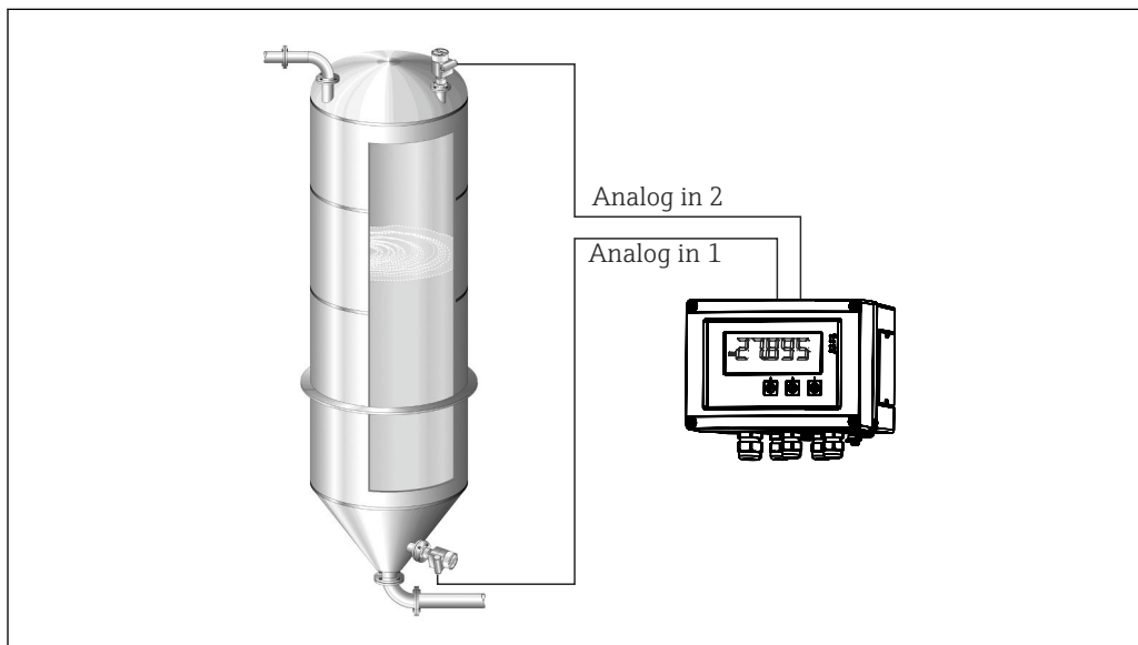
8 Применение для измерения дифференциального давления
