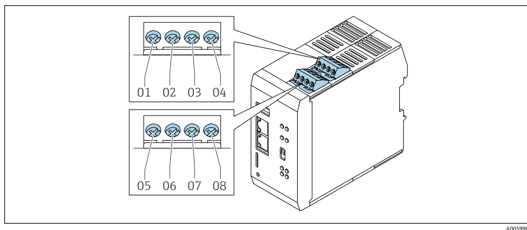
图 34 脉冲输入和模拟量输入
