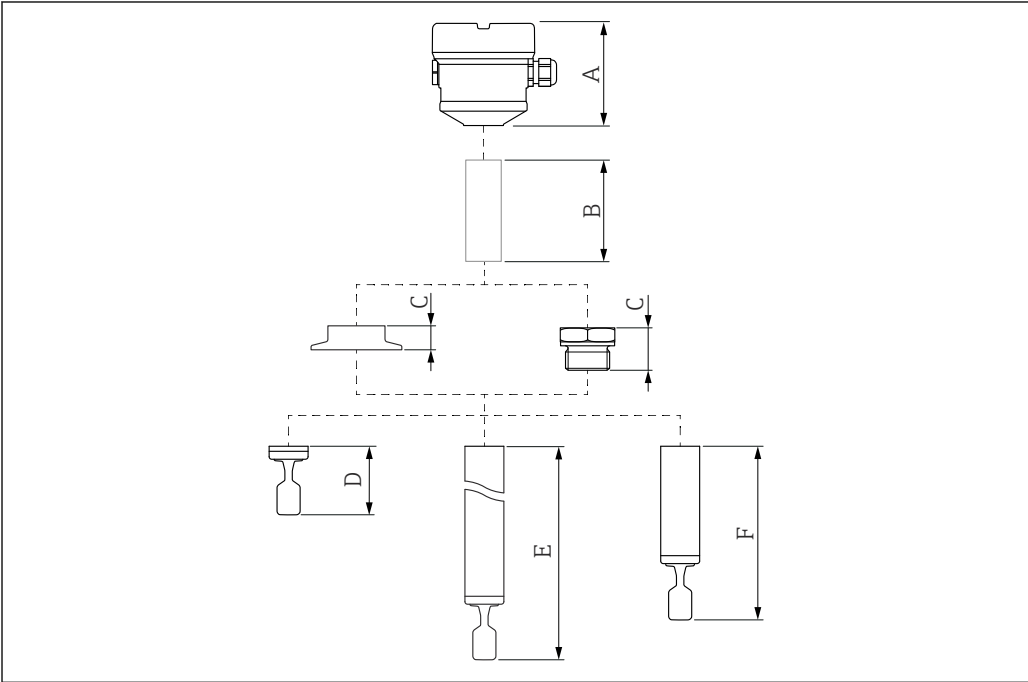
图 13 计算仪表高度所需考虑的部件
