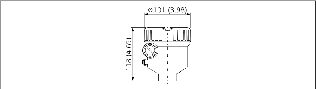
16 单腔体铝外壳（带涂层）的外形尺寸示意图；适用 Ex d/XP、粉尘防爆场合；外壳盖不带观察窗。测量单位 mm (in)
