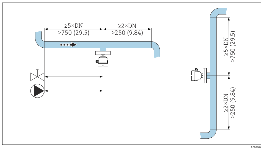
图 5 前直管段的安装。测量单位 mm (in)
