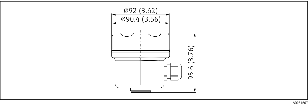
17 单腔体 316L 外壳（卫生型）的外形尺寸示意图；外壳盖不带观察窗。测量单位 mm (in)
