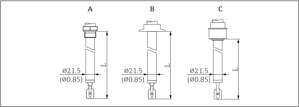
图 20 探头类型：延长管型、短管型（传感器长度 L）。测量单位 mm (in)
