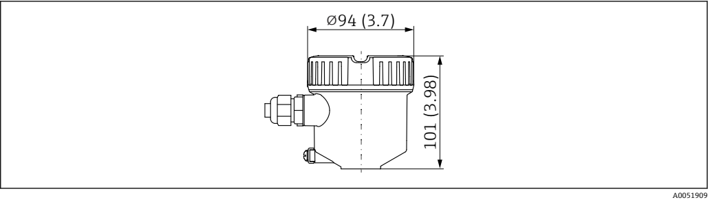
14 单腔体塑料外壳的外形尺寸示意图；外壳盖不带观察窗。测量单位 mm (in)
