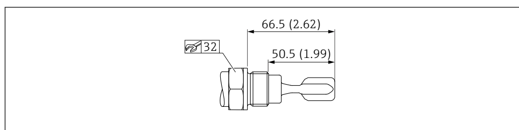
图 23 ISO228 G 3/4 螺纹。测量单位 mm (in)
