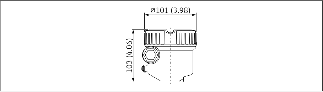
15 单腔体铝外壳的外形尺寸示意图；外壳盖不带观察窗。测量单位 mm (in)
