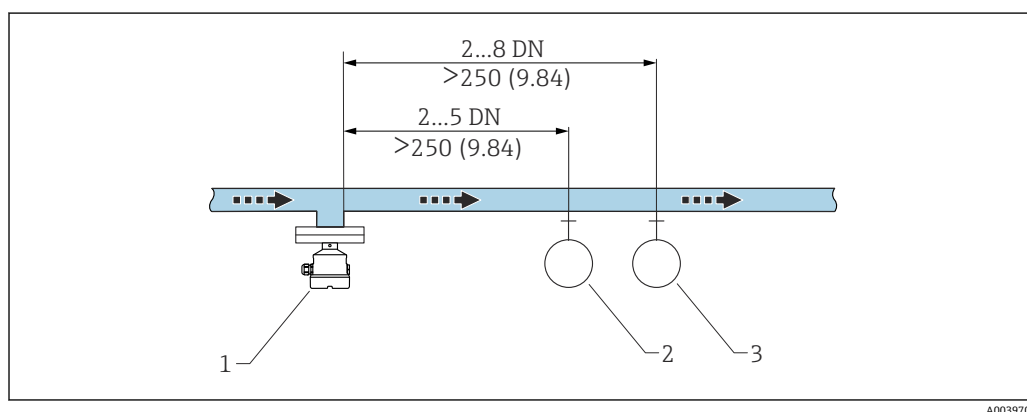
图 6 后直管段的安装。测量单位 mm (in)
