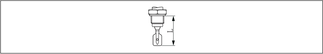
图 19 探头类型：一体式；传感器长度 L
