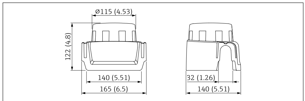
30 Защитный козырек для однокамерного корпуса из алюминия. Единица измерения мм (дюйм)
