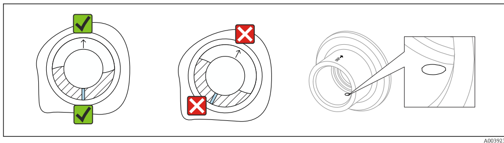
10 Сварной переходник с отверстием для утечек
