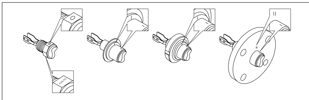
11 Положение вибрационной вилки при горизонтальном монтаже в резервуаре с помощью маркировки
