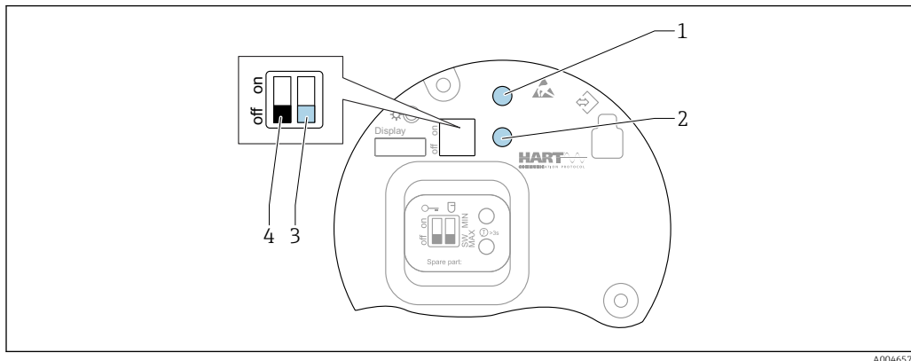
26 Кнопки управления и DIP-переключатель на электронной вставке FEL60H
