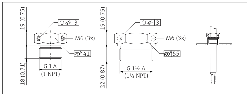
32 Скользящие муфты для использования при отсутствии избыточного давления, p_e = 0 бар (0 фунт/кв. дюйм). Единица измерения мм (дюйм)
