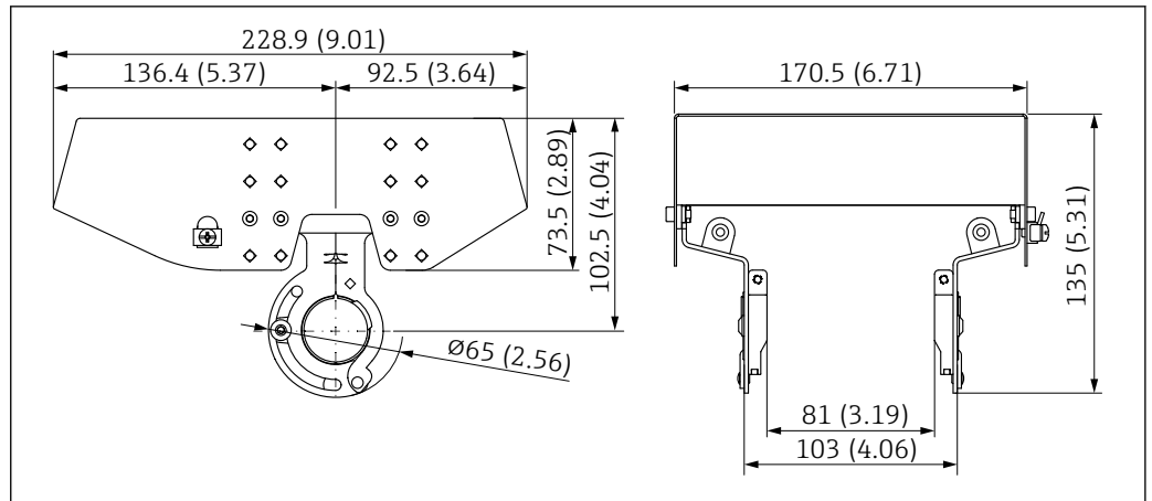
29 Защитный козырек от погодных явлений для корпуса с двумя отсеками. Единица измерения мм (дюйм)
