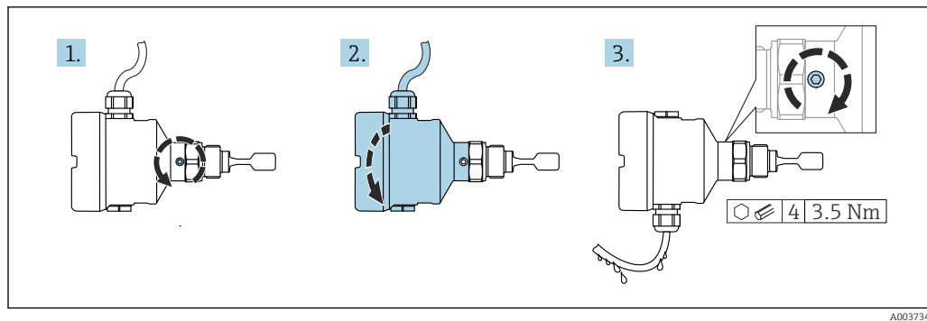
15 Корпус с наружным стопорным винтом и ниспадающей каплеуловительной кабельной петлей
