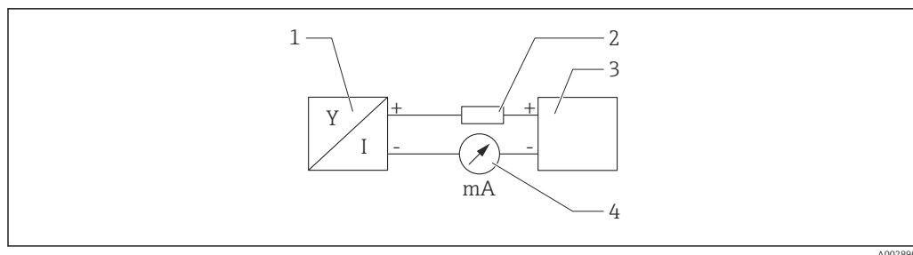
17 Блок-схема подключения HART
