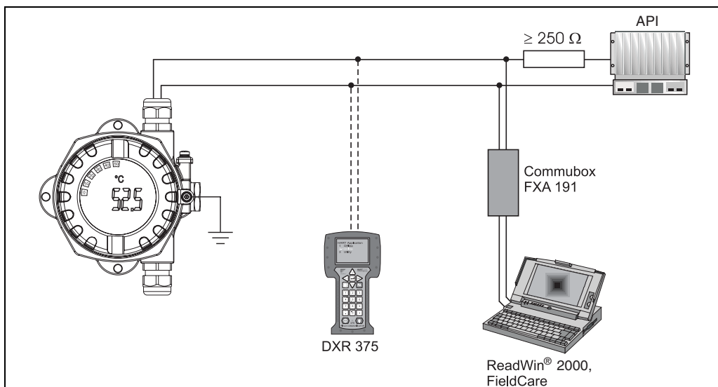
fig. 7 : Raccordement HART® avec d'autres alimentations
