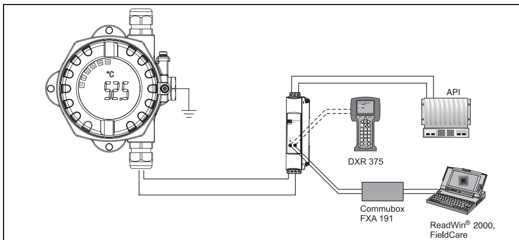
fig. 6 : Raccordement HART® avec alimentation E+H RN 221N
