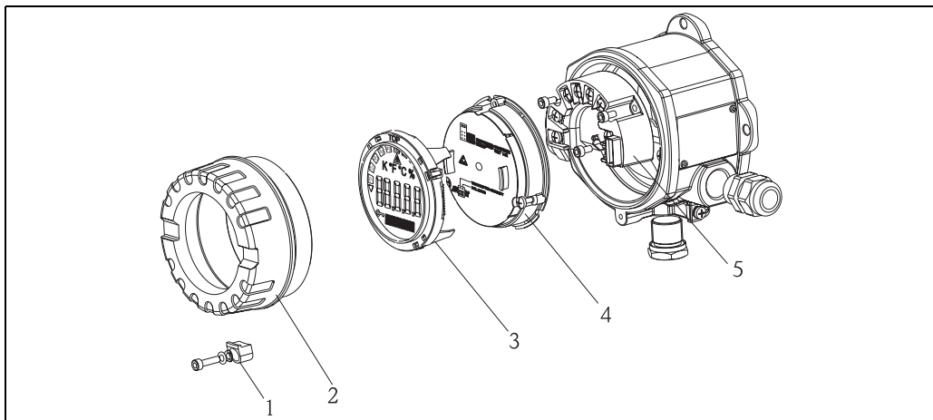
fig. 3 : Orientation de l'afficheur
