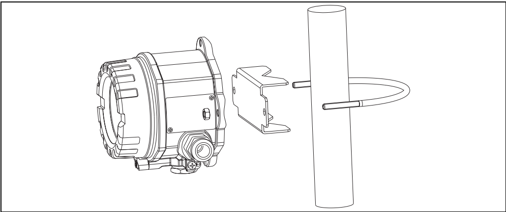
Abb. 4: Montage des Feldtransmitters mit Montagehalter, siehe Kap. 'Zubehör'
