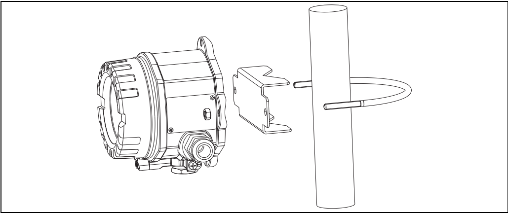
fig. 4 : Montage du transmetteur de terrain avec étrier, voir chap. 'Accessoires'
