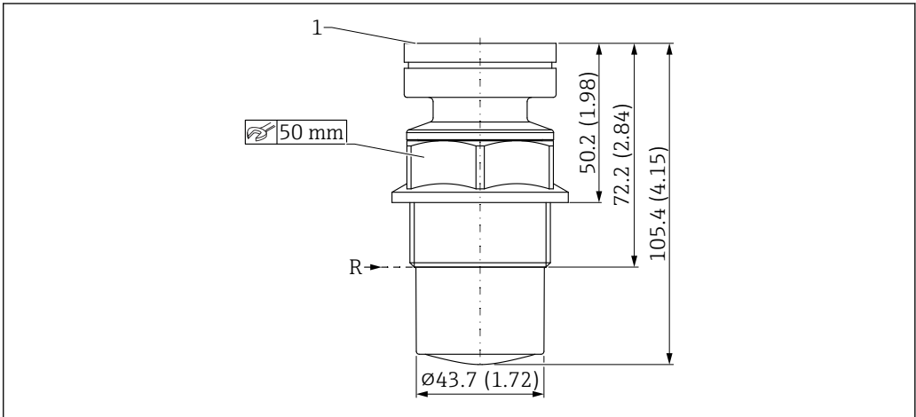
46 PVDF 全密封天线 (40 mm (1.5 in) 口径) 的外形尺寸示意图。测量单位 mm (in)
