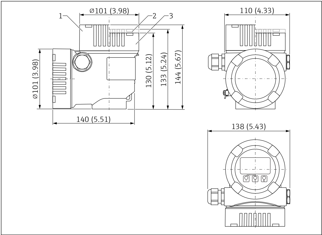
45 L 型双腔室 316L 外壳的外形尺寸示意图；包括 M20 接头和塑料插头。测量单位 mm (in)
