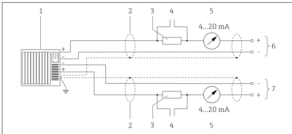
10 Esempio di connessione per l'ingresso HART (modalità di master) mediante l'uscita in corrente (attiva)
