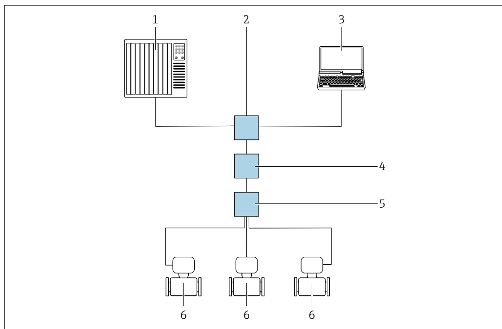
图 15 通过 Modbus TCP + Ethernet-APL 通信进行远程操作（有源信号）
