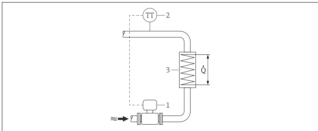
6 蒸汽和水热量差值测量示意图
