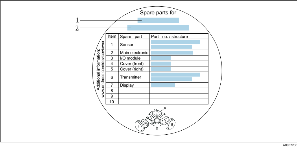
图 21 接线腔盖中的“备件标签”示例
