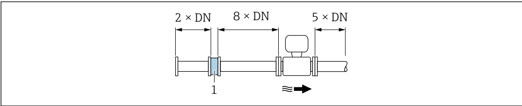
1 流量调节器
