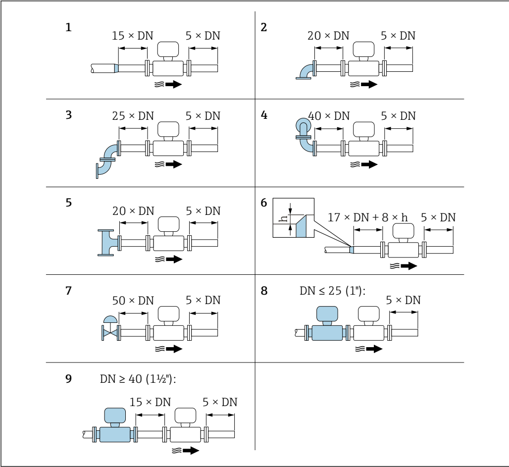
图 4 使用不同节流装置时的最小前后直管段长度
