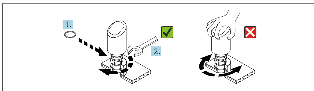
13 Вворачивание прибора
