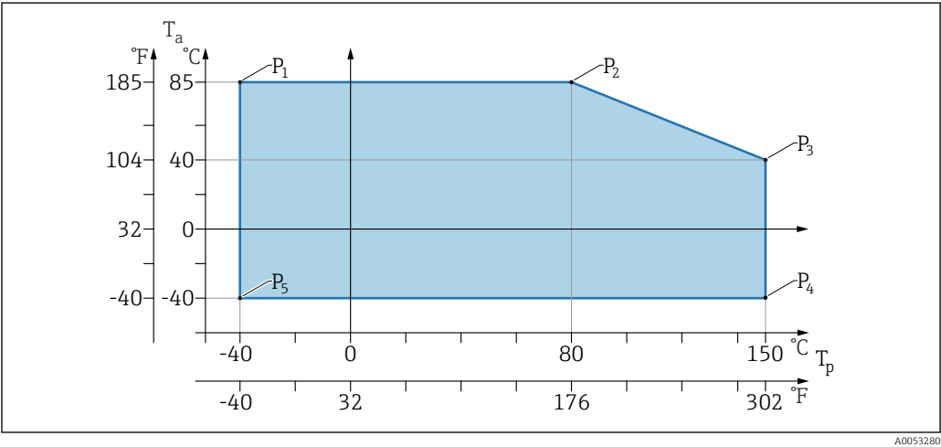
22 Зависимость температуры окружающей среды T_a от рабочей температуры T_p
