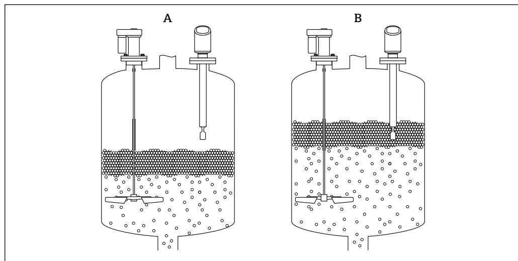
20 Функциональность опции "Обнаружение пены"
