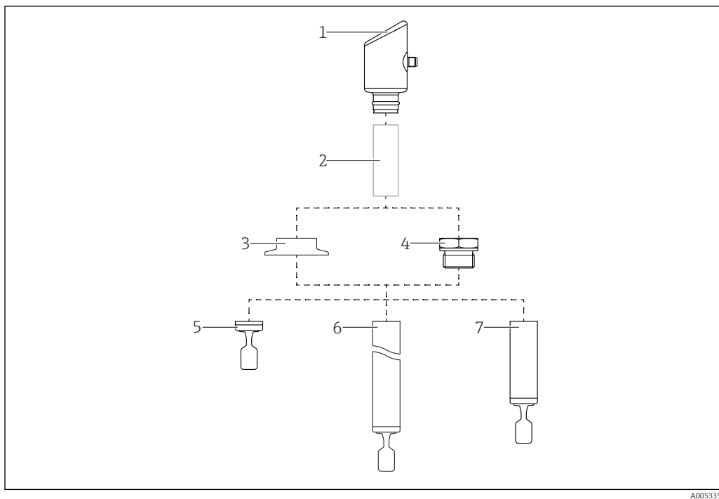
1 Конструкция изделия
