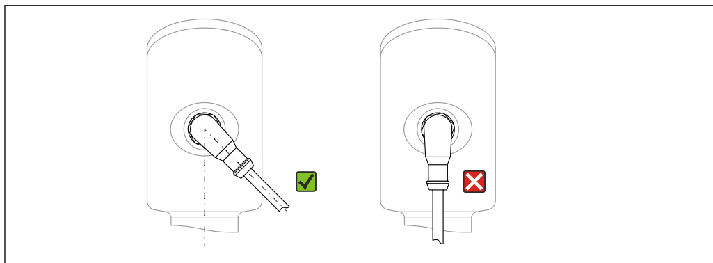
15 Выравнивание разъема M12
