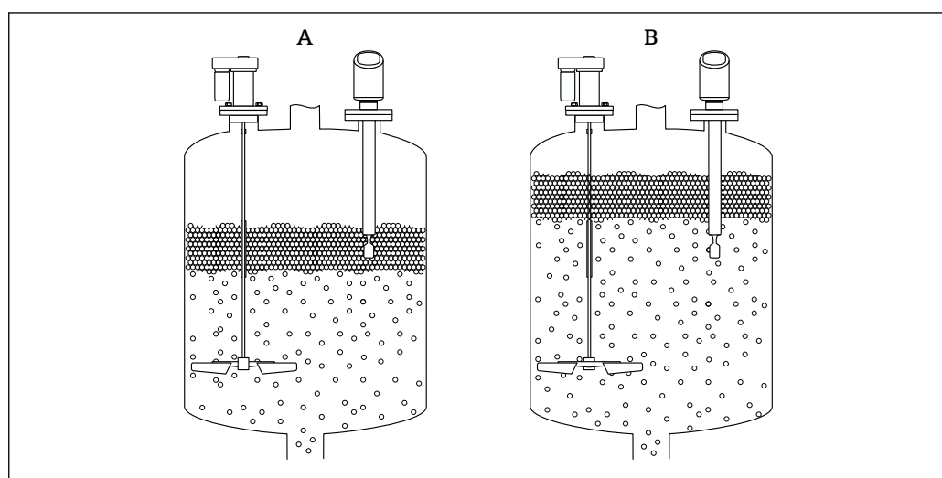
21 Функциональность опции "Игнорировать пену"
