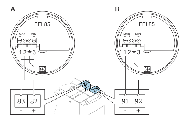
3 Připojení ke svorkovnicím nahore, příklad senzoru FEL85
