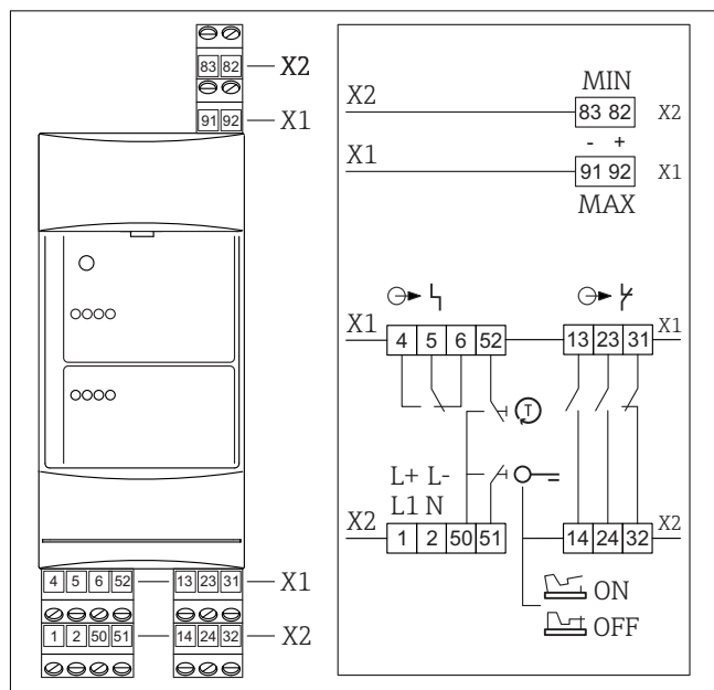
2 Čelní panel otevřený, připojení ke svorkovnicím
