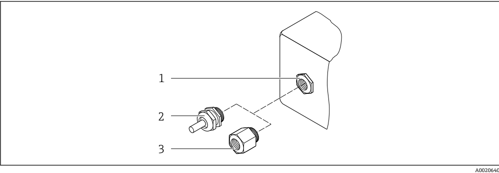
図 43 可能な電線口/ケーブルグランド 1 めねじ M20 × 1.5 2 ケーブルグランド M20 × 1.5 3 電線口用アダプタ（めねじ G ½" または NPT ½"）
