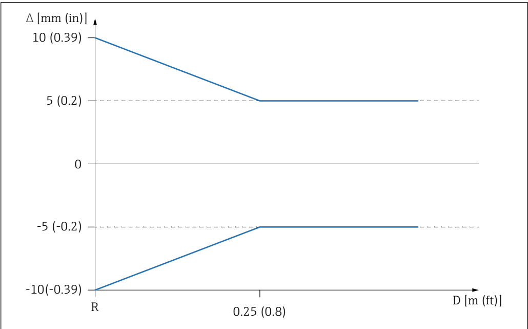
4 Écart de mesure maximal dans la portée proximale
