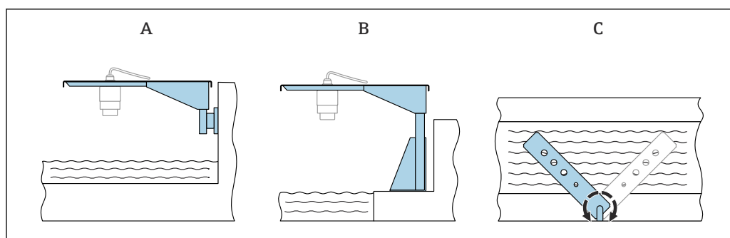
■ 13 Montage avec bras de montage, avec pivot
