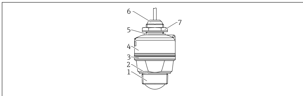
■ 18 Aperçu des matériaux ; antenne 40 mm (1,5 in), filetage entrée de câble
