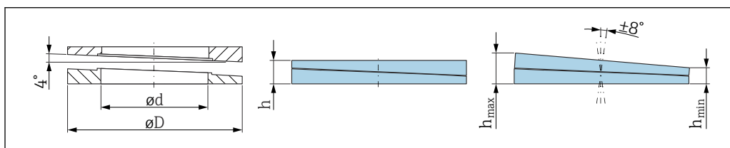
45 Dimensions
