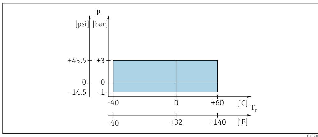
15 Gamme autorisée pour la température et la pression de process
