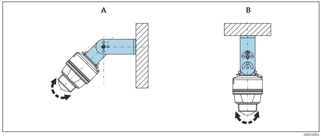
11 Montage avec un étrier de montage réglable
