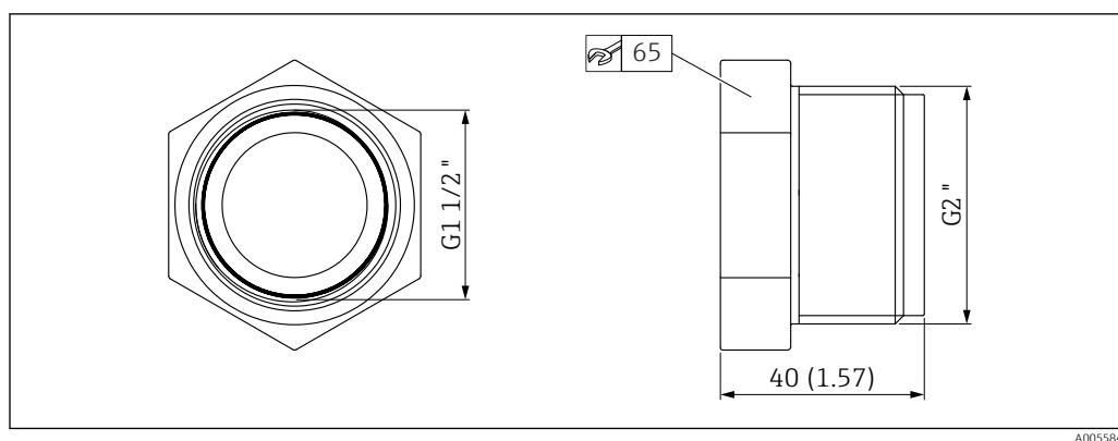
23 Dimensions de l'adaptateur UNI
