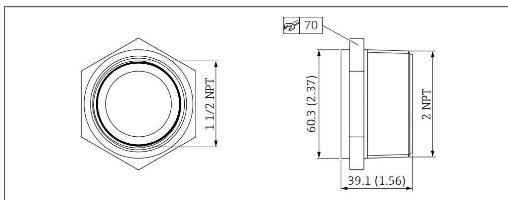
24 Dimensions de l'adaptateur UNI
