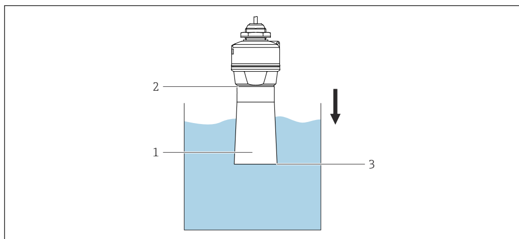
10 Principe de fonctionnement du tube de protection antidébordement
