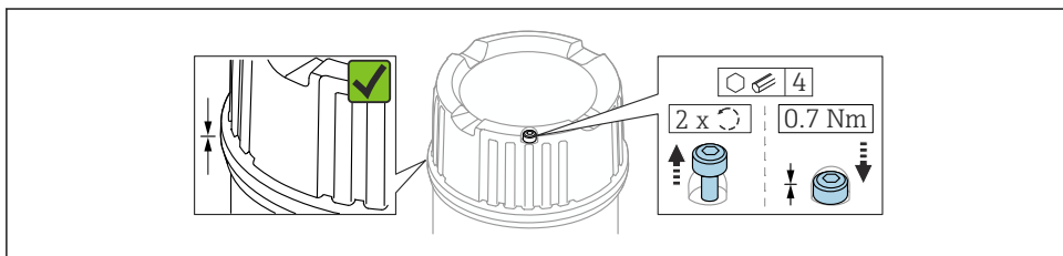
15 带锁定螺丝的外壳盖
