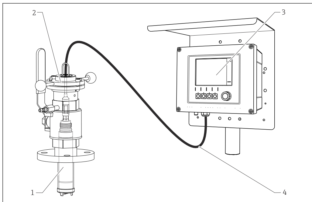
图 6 测量系统示例，连接 Memosens COS51E 数字式溶解氧传感器
