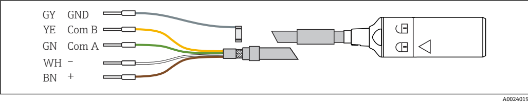
图 18 测量电缆，例如 CYK10 或
