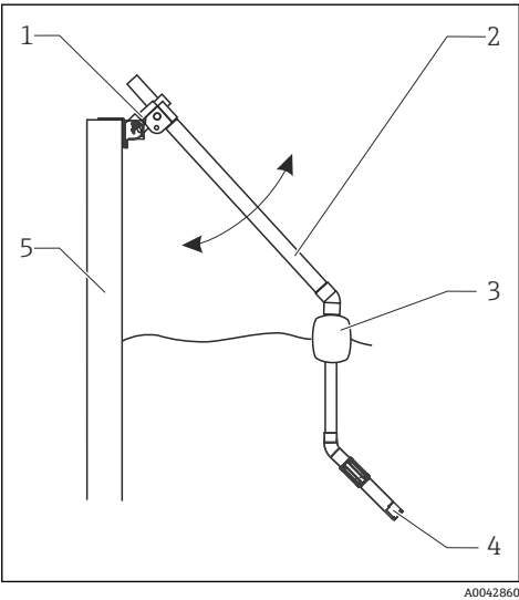
图 11 池边安装
