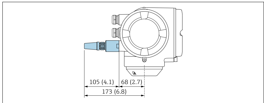
■ 32 Unidad mm (in)
