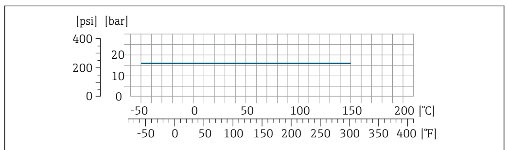
23 Con material de conexión titanio de grado 2
