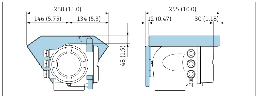
26 Unidad mm (in)
