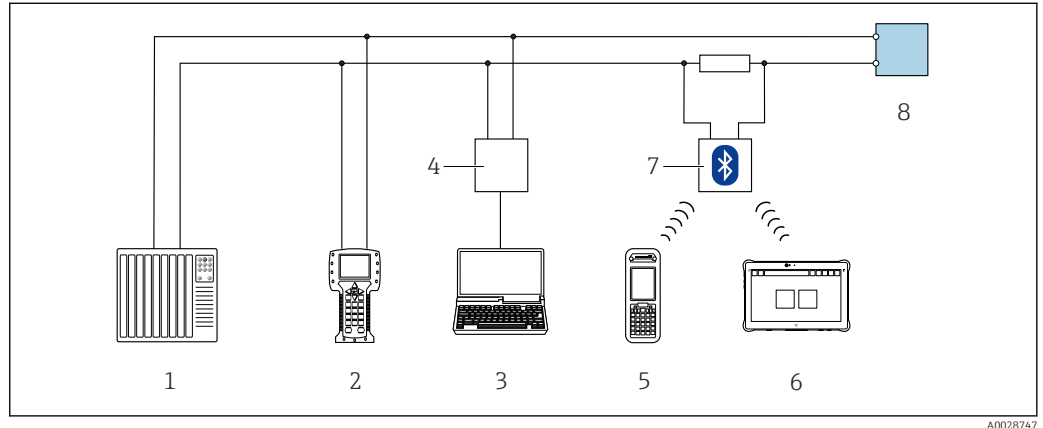
37 Opciones para la configuración a distancia mediante el protocolo HART (activo)
