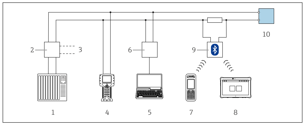
38 Opciones para la configuración a distancia mediante el protocolo HART (pasivo)
