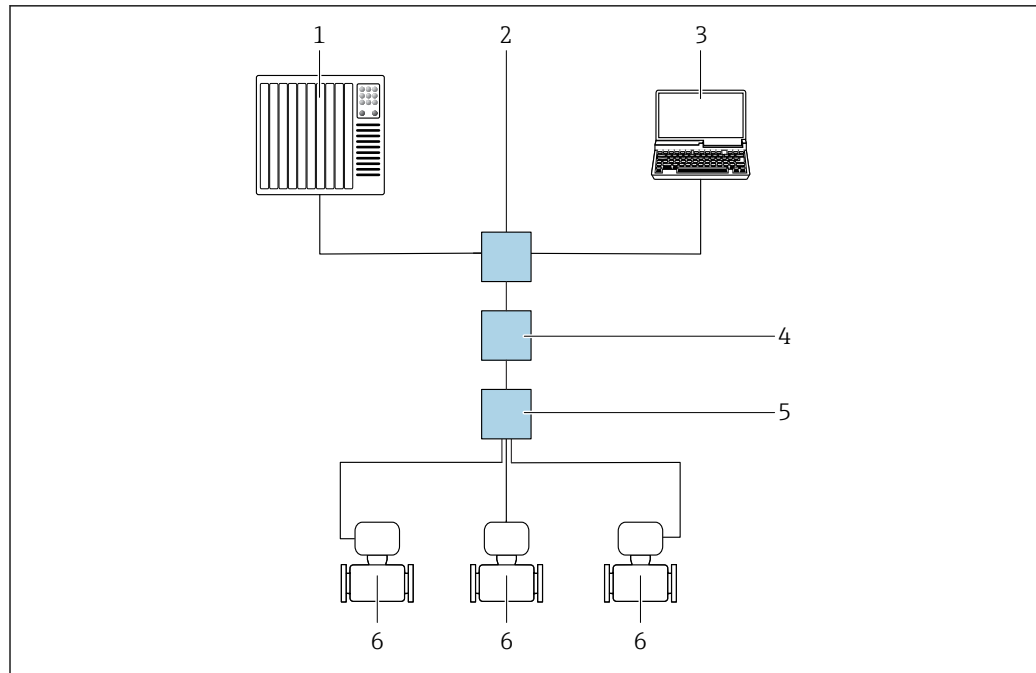
43 Opciones de configuración a distancia mediante el protocolo Modbus TCP a través de Ethernet-APL (activo)
