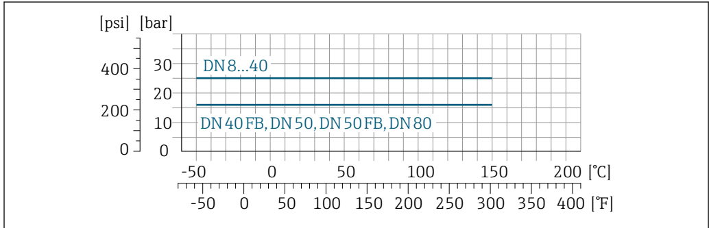
19 Con material de la brida titanio de grado 2
