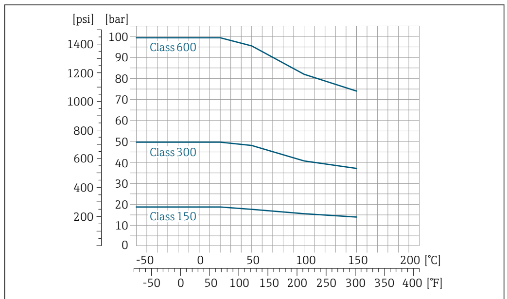
17 Con material de la brida 1.4301 (304); partes en contacto con el producto: titanio
