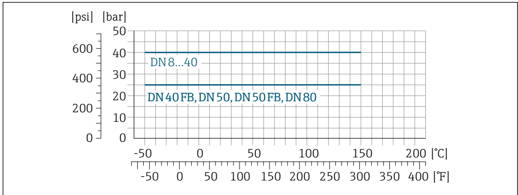
20 Con material de conexión titanio de grado 2
