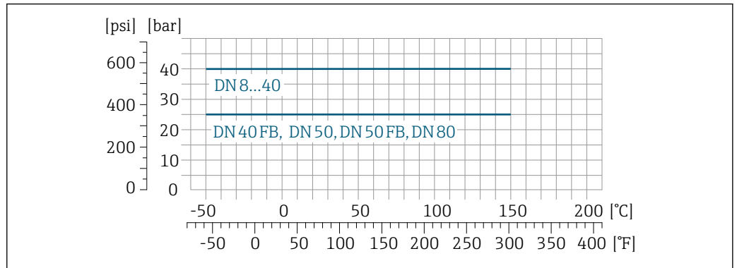
21 Con material de conexión titanio de grado 2
