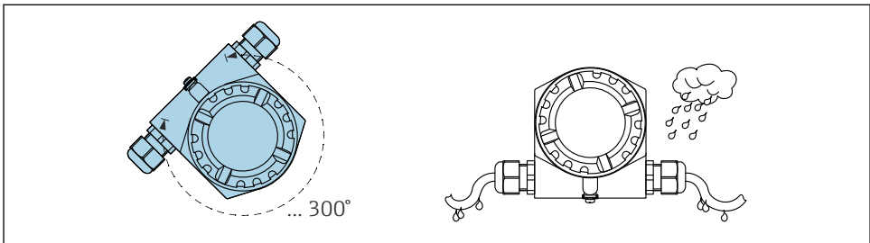
15 Boîtier sans vis de réglage ; former une boucle de drainage sur le câble
