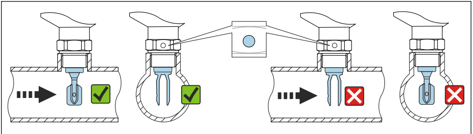
12 Montage dans des conduites (tenir compte de la position de la fourche et du marquage)
