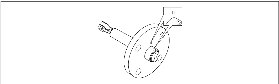
11 Positionner la fourche vibrante lors d'un montage horizontal dans la cuve à l'aide du marquage
