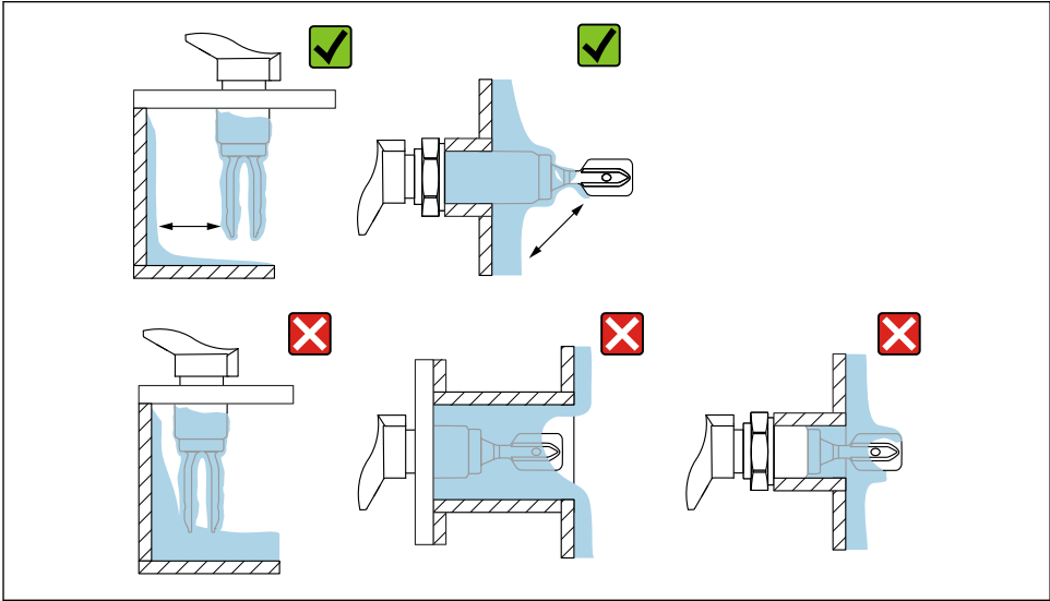
8 Exemples de montage pour un produit de process fortement visqueux
