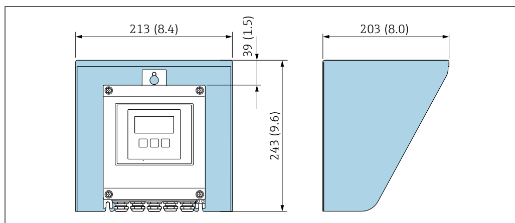
39 Capot de protection climatique pour Proline 500 – numérique ; unité mm (in)
