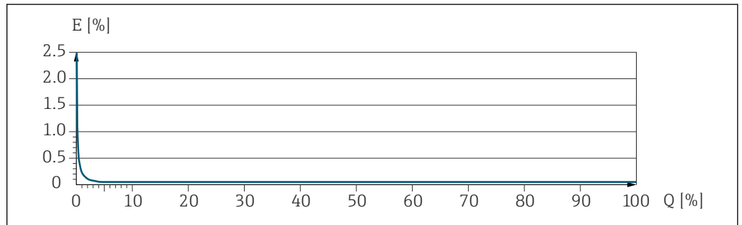
E Écart de mesure maximal en % de m. (exemple avec PremiumCal) Q Débit en % de la valeur de fin d'échelle maximale
