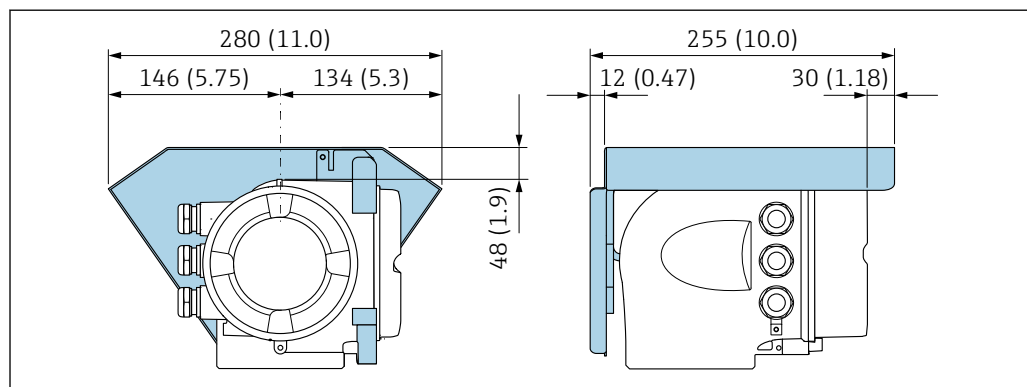
40 Capot de protection climatique pour Proline 500 – unité mm (in)
