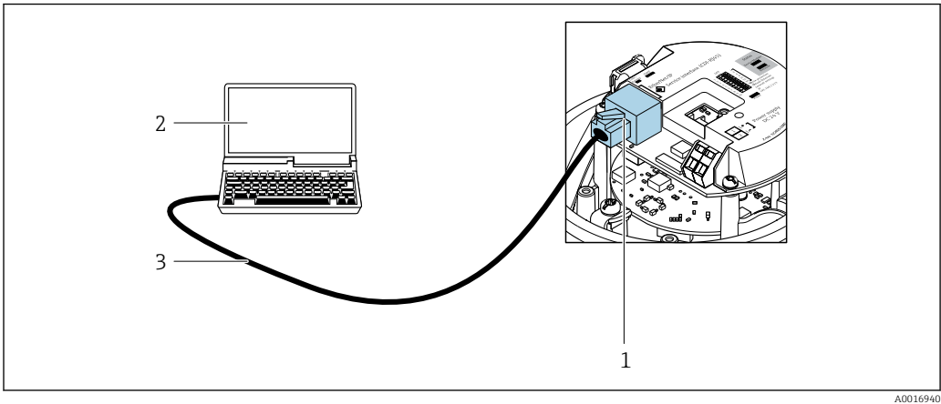
18 Connexion pour la caractéristique de commande "Sortie", option R : PROFINET 1 Interface service (CDI-RJ45) et interface Profinet de l'appareil de mesure avec accès au serveur web intégré 2 Ordinateur avec navigateur web pour l'accès au serveur web intégré ou avec outil de configuration FieldCare et COM DTM "CDI Communication TCP/IP" 3 Câble de raccordement Ethernet standard avec connecteur RJ45
