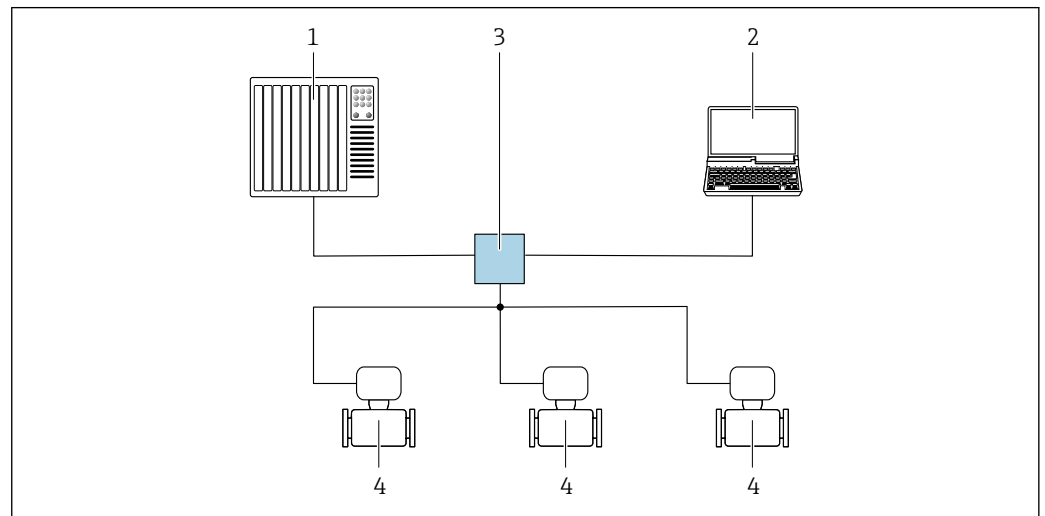
17 Options de configuration à distance via réseau PROFINET : topologie en étoile
