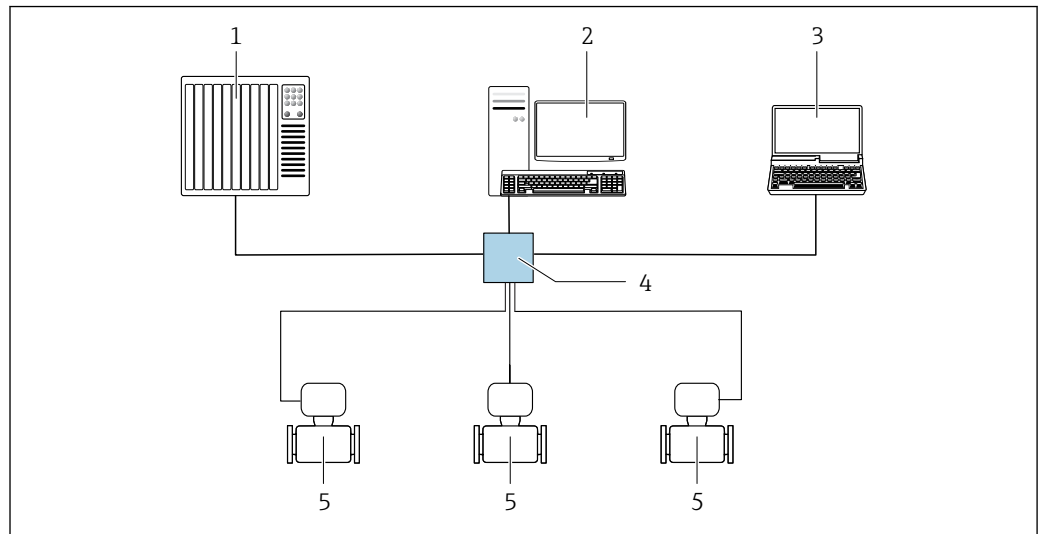
31 Opções para operação remota através do Modbus TCP por Ethernet - 100 Mbit/s: Topologia estrela
