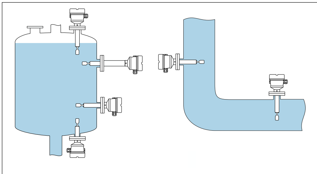
4 Примеры монтажа в резервуаре, баке или трубопроводе
