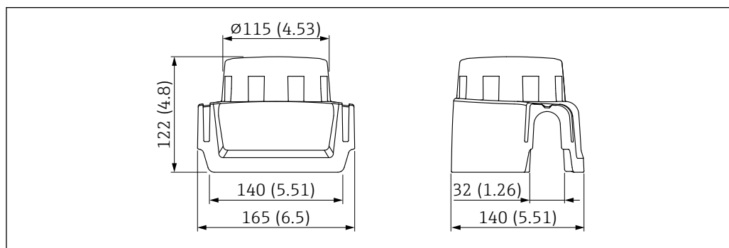
24 Защитная крышка для алюминиевого корпуса с одним отделением. Единица измерения мм (дюйм)
