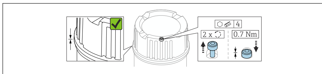
18 Крышка с крепежным винтом
