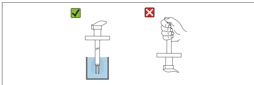
22 Функциональное испытание вибрирующей вилки
