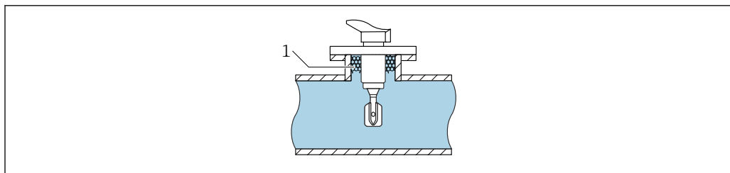
6 Пример монтажа в потоке технологической среды в трубопроводах
