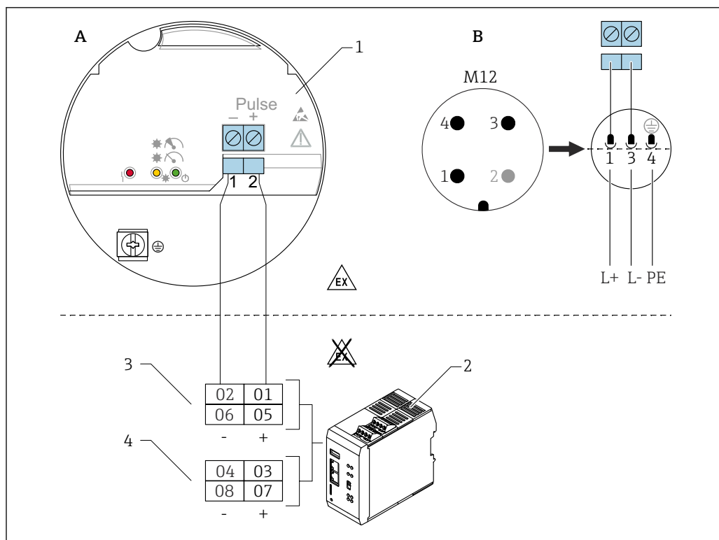
19 Схема подключения электронной вставки FEL60D к вычислителю плотности Density Computer QML51
