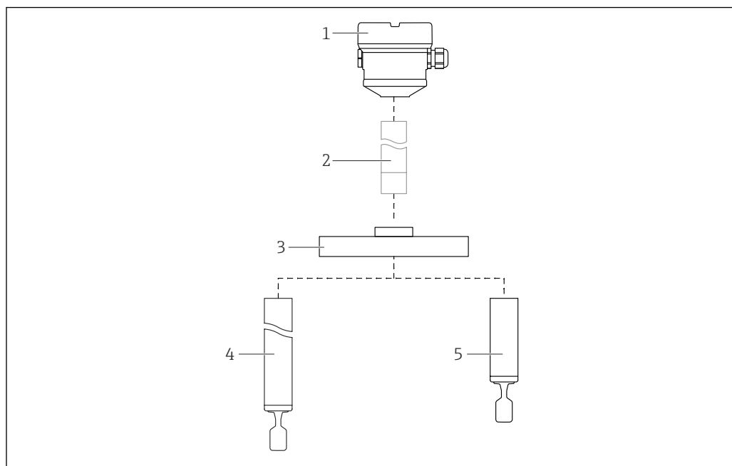
2 Конструкция изделия Liquiphant FTL62
