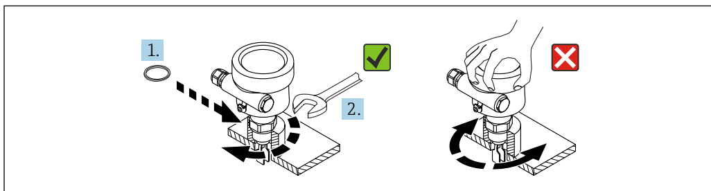
15 Прикручивание прибора
