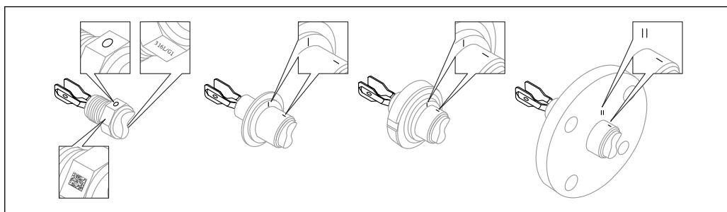
13 Положение вибрационной вилки при горизонтальном монтаже в резервуаре с использованием маркировки
