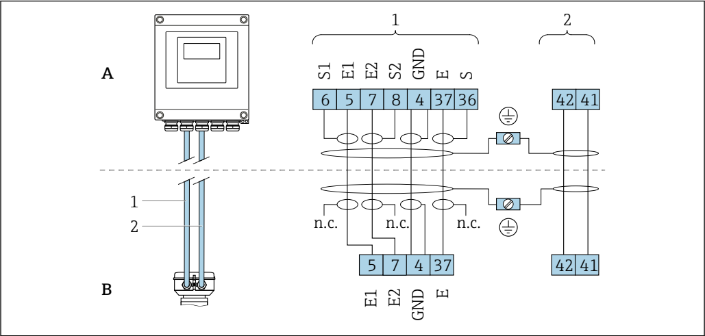
图 9 分体型仪表的接线端子分配 A 变送器的墙装外壳 B 传感器接线盒 1 电极电缆 2 供电电缆 n.c. 悬空不连接，电缆屏蔽层绝缘处理
