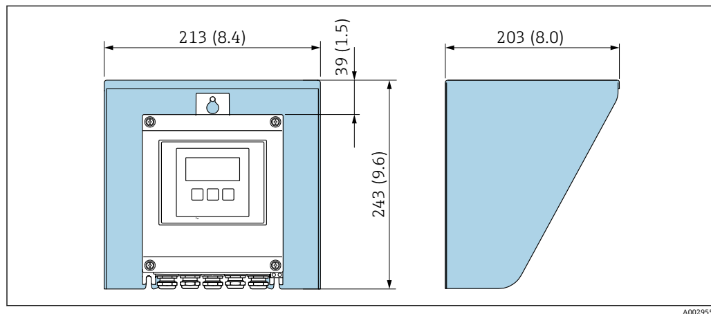
图 4 防护罩的外形尺寸示意图；单位：mm (in)
