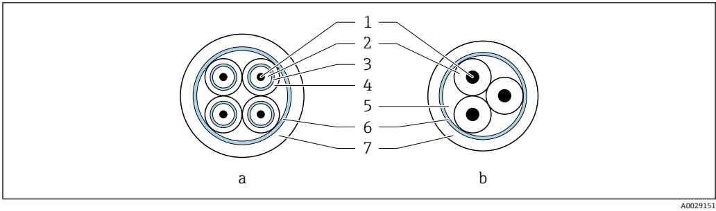
8 电缆截面图
