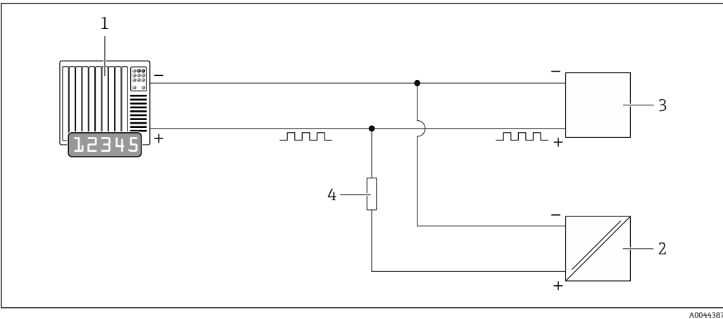
图 15 接线实例：脉冲输出（无源信号）
