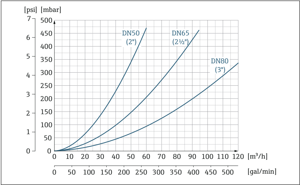
18 压损: 适用口径 DN 50...80 (2...3"); 订购选项“设计”, 选型代号 C “固定法兰, 缩径测量管, 无前后直管段长度要求”
