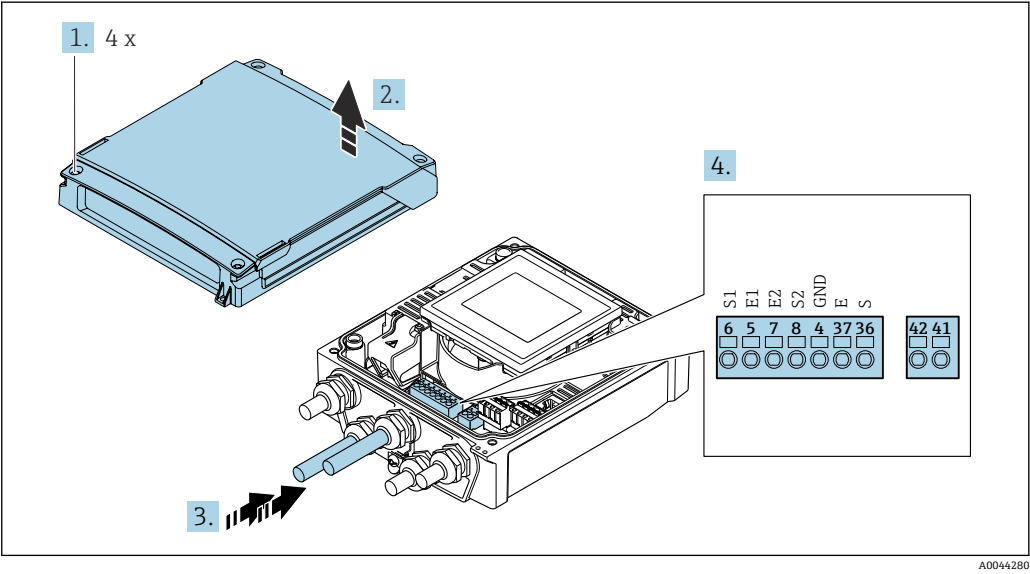
图 13 变送器：带接线端子的主要电子模块
