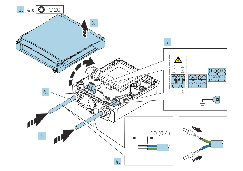
14 连接电源
