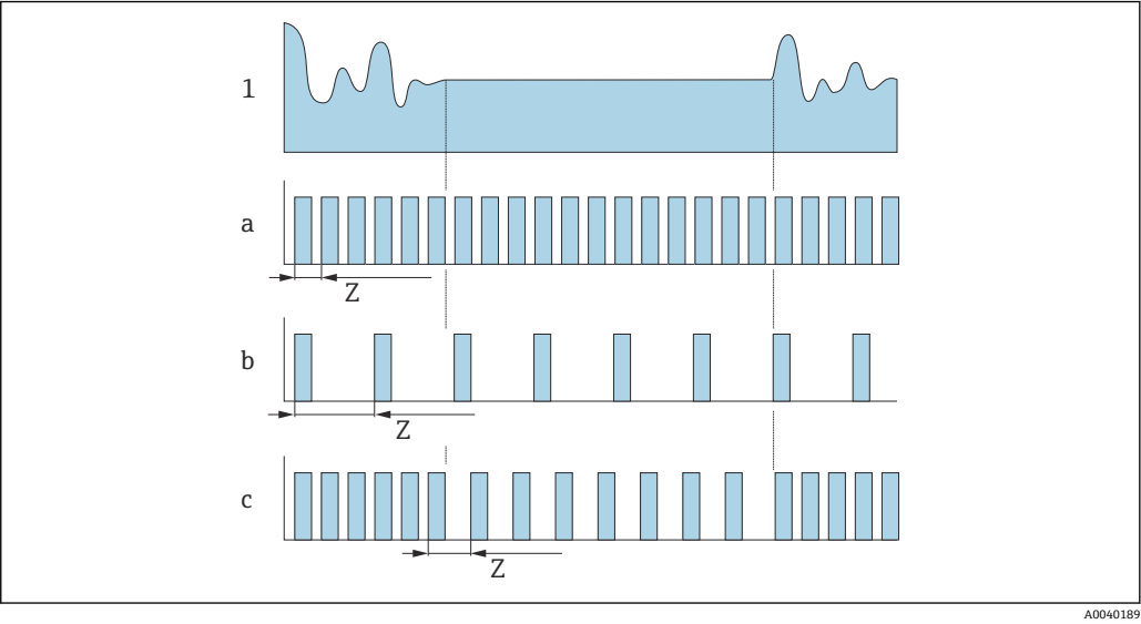
16 不同数据记录方式的工作原理
