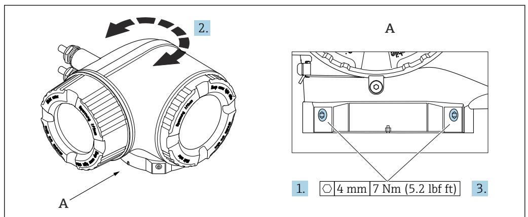
■ 6 防爆型外壳
