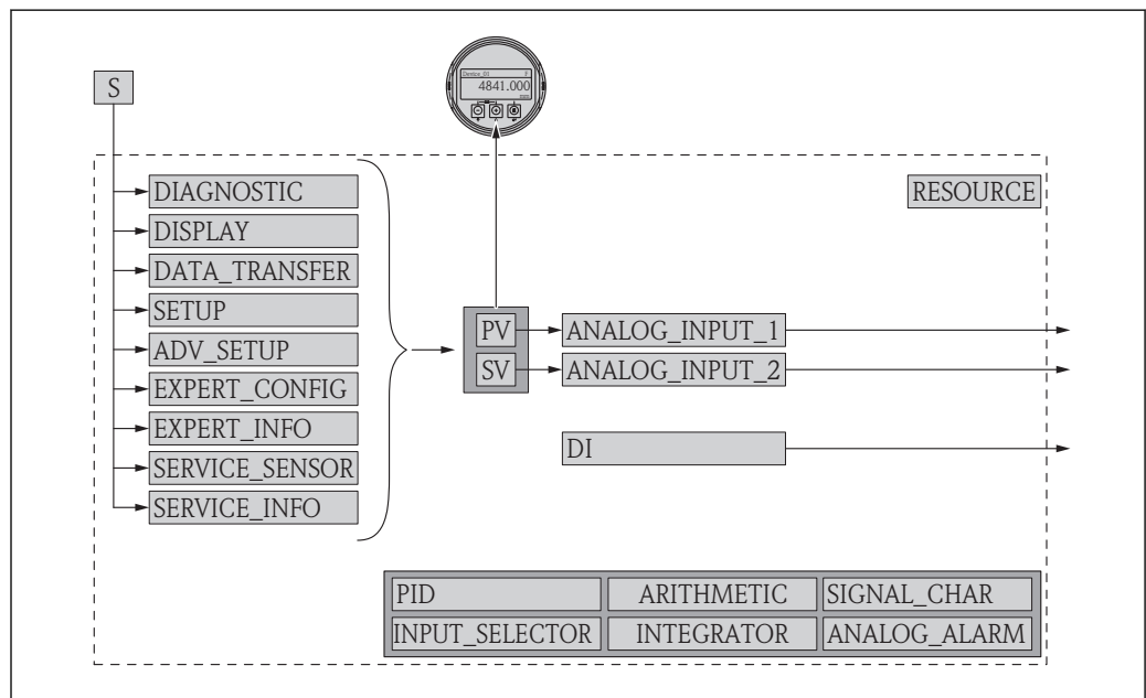
16 Configuration des blocs à la livraison
