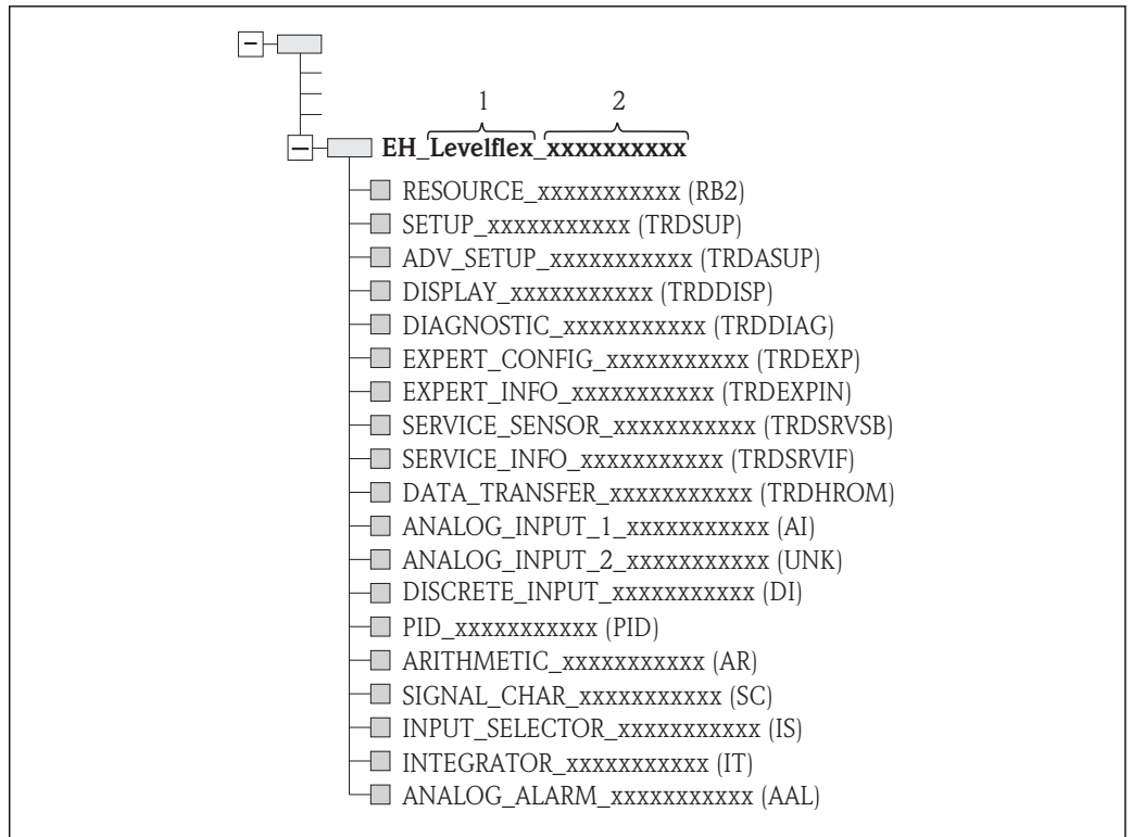
15 Représentation typique dans un logiciel de configuration après l'établissement de la connexion
