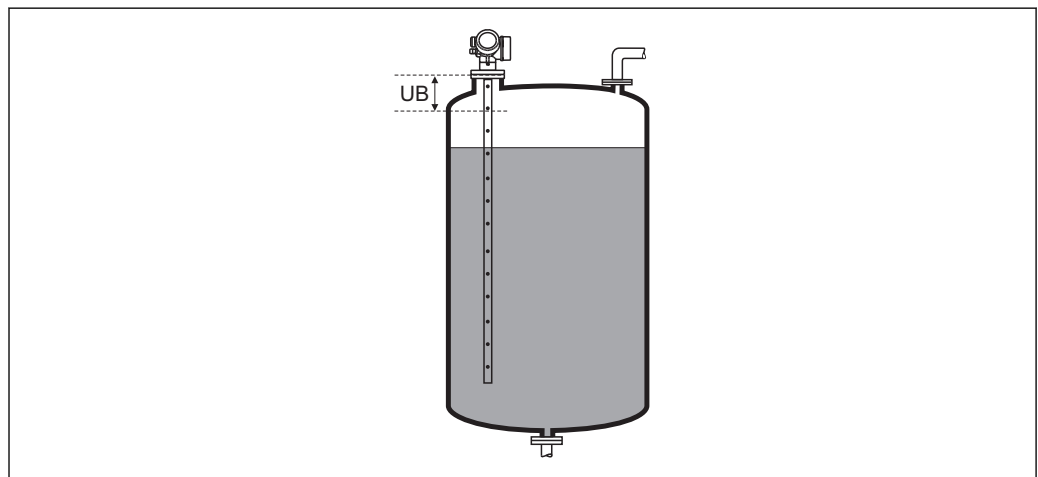
📄 33 Distance de blocage (UB) pour la mesure dans les liquides
