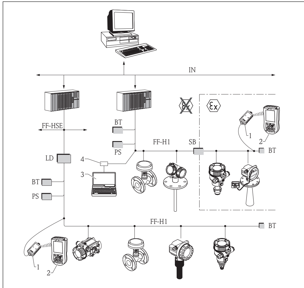
13 Architecture du système FOUNDATION Fieldbus avec composants associés
