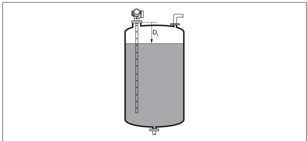
☰ 32 Distance pour la mesure sur liquides
