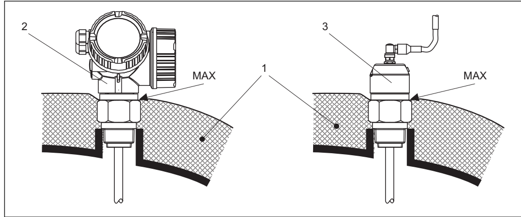
6 Raccord process avec filetage - FMP50
