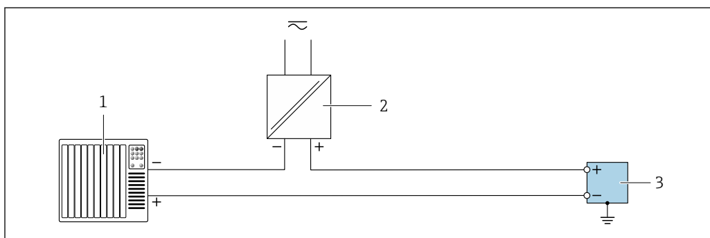
7 Пример подключения для импульсного/частотного/релейного выхода (пассивного)
