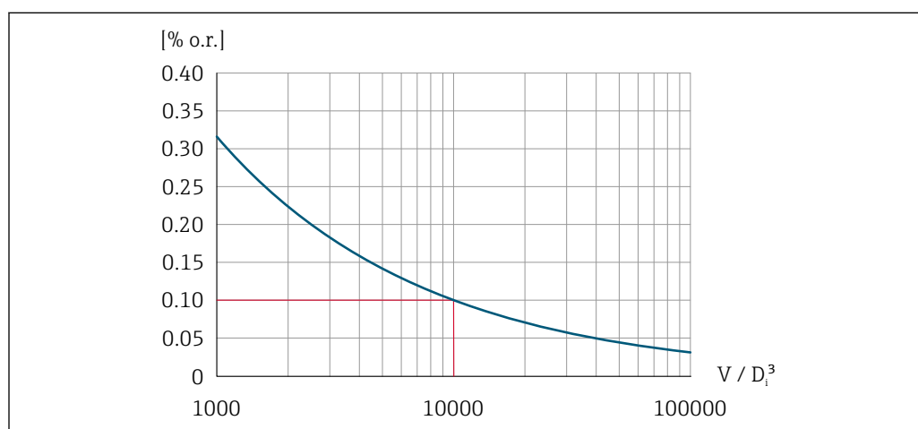
10 Повторяемость – 0,1 % ИЗМ при измерении объемного расхода ( m^3 ) от V = 10000 \cdot D_i^3
