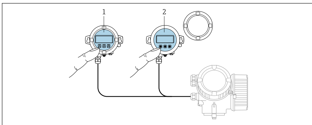
20 Варианты управления FHX50
