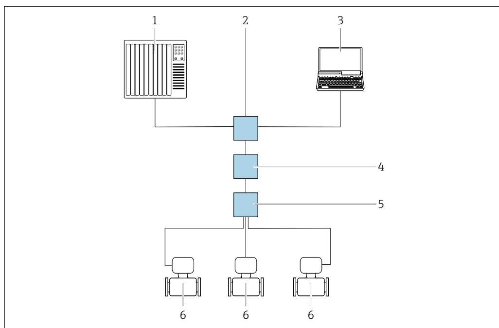
24 Варианты дистанционного управления через протокол Modbus TCP через Ethernet-APL (активный)
