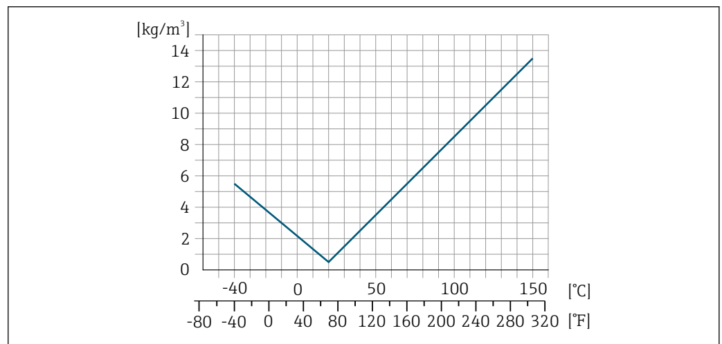
43 Felddichtejustierung, Beispiel bei +20 °C (+68 °F)
