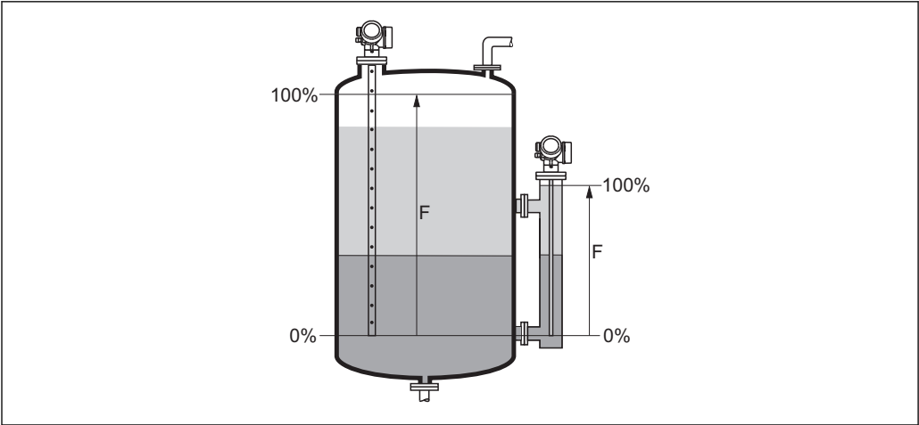
16 Abgleich Voll (F) bei Trennschichtmessungen
