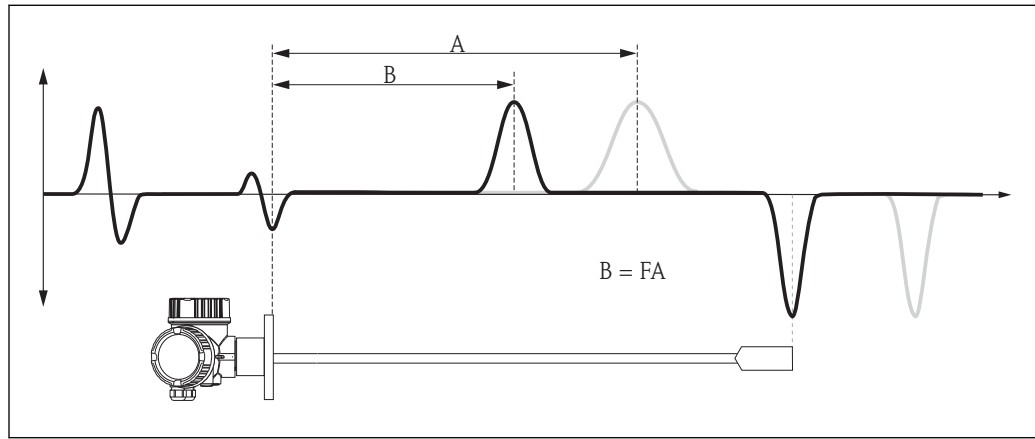
34 Gasphasenkompensation mit konstantem Kompensationsfaktor F
