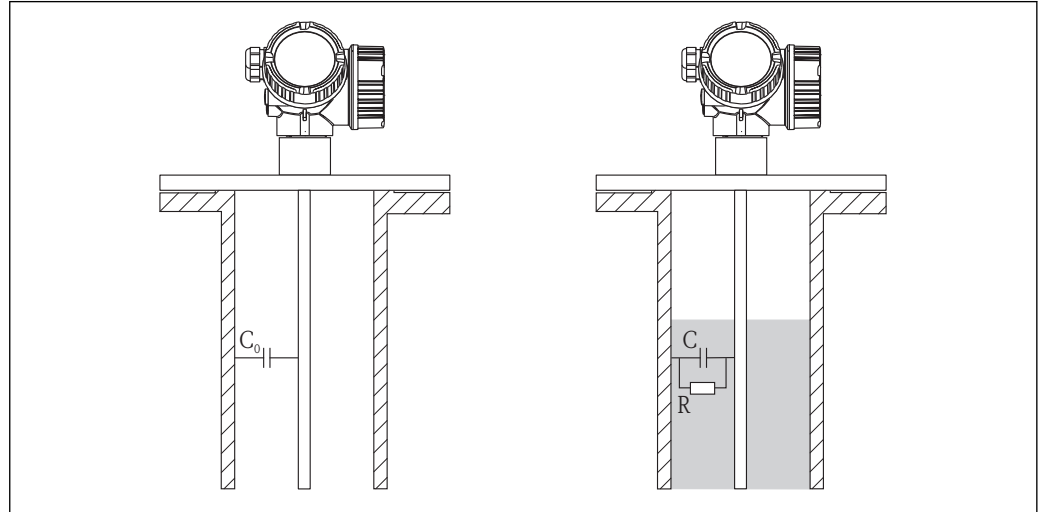
52 Kapazitive Füllstandmessung
