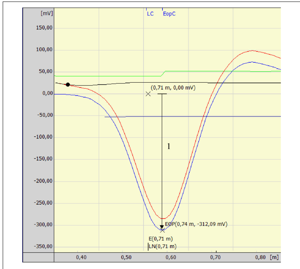
1 Absolute EOP-Amplitude (Beispiel für isoliertes Sondenende)
