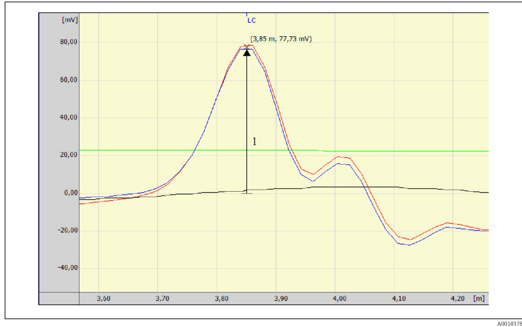
1 Absolute Echoamplitude in der Hüllkurve, gemessen von der 0mV-Linie
