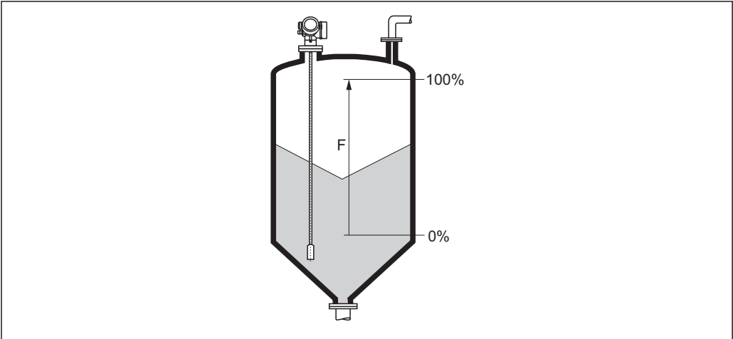
17 Abgleich Voll (F) bei Messungen in Schüttgütern
