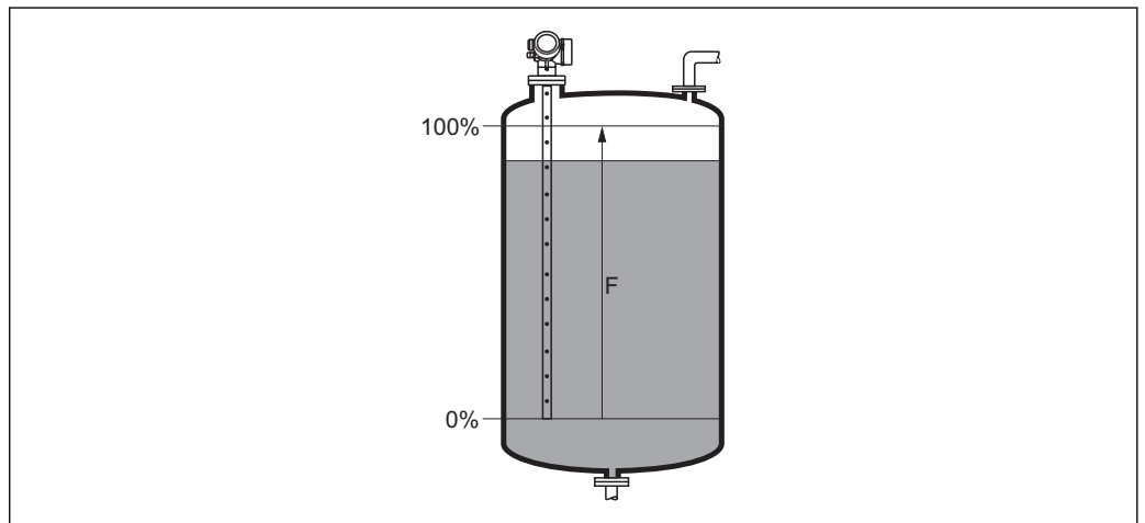
15 Abgleich Voll (F) bei Messungen in Flüssigkeiten
