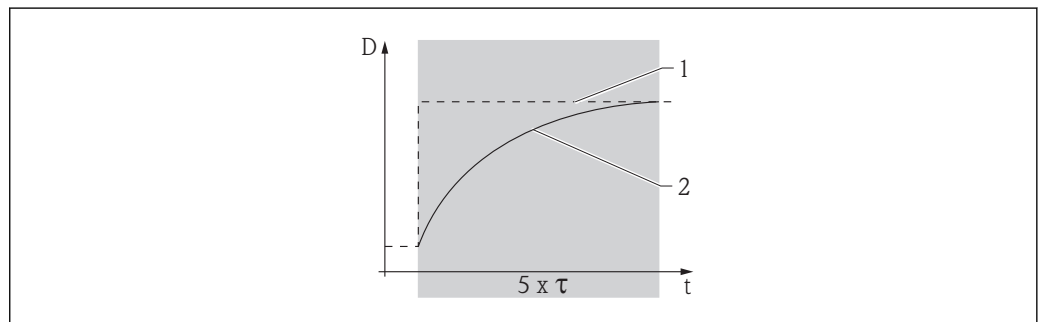
26 Tiefpassfilter
