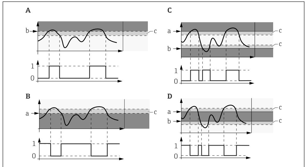
59 Grenzwertüberwachung im Erweiterte-Diagnose-Block
