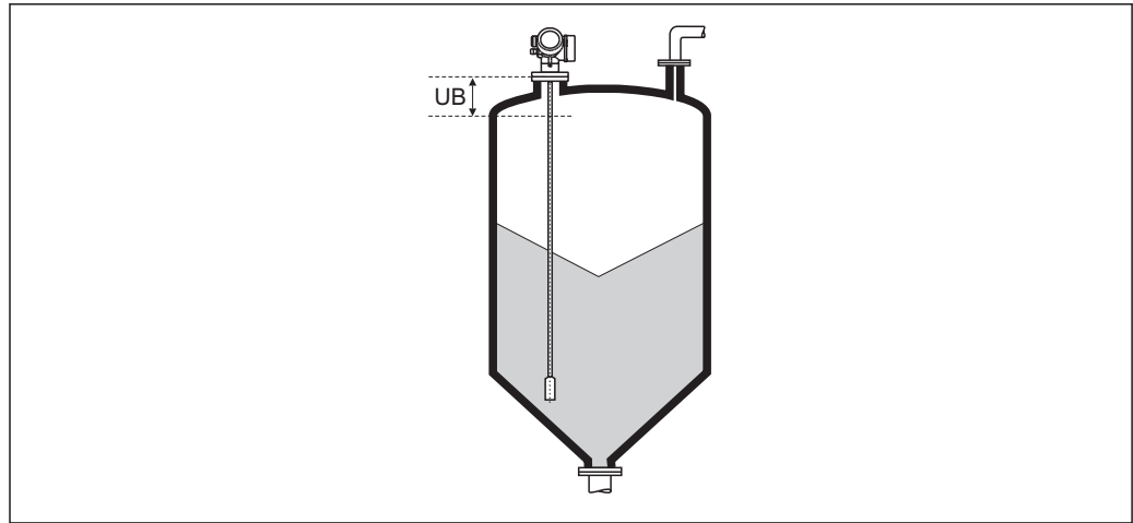
32 Blockdistanz (UB) bei Messung in Schüttgütern
