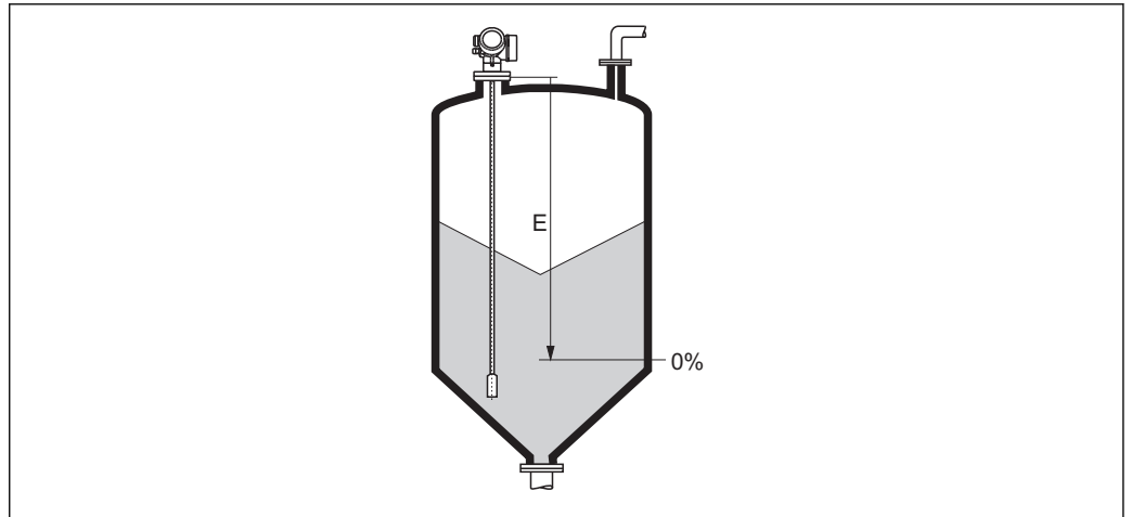
14 Abgleich Leer (E) bei Messungen in Schüttgütern
