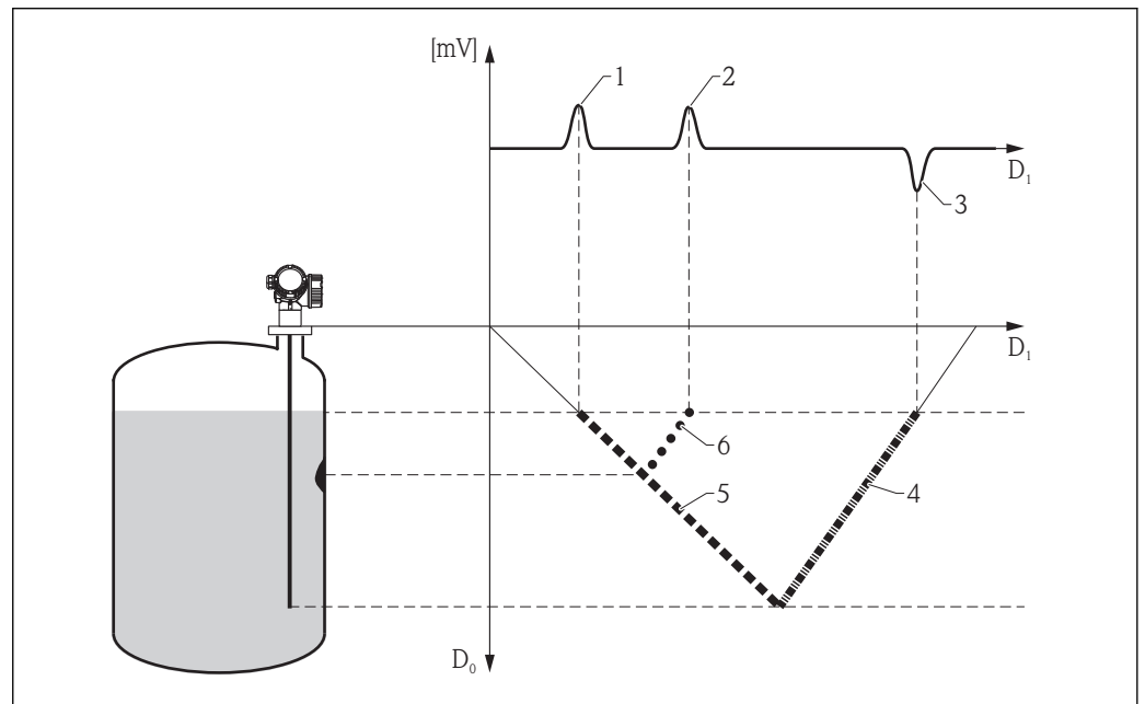
49 Beispiel 1: Tankhistorie mit Störecho und Sondenendecho (kleiner DK-Wert)
