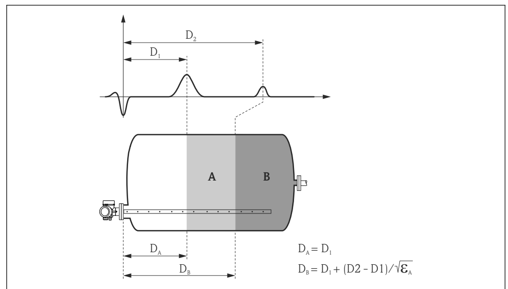
51 Trennschichtmessung mit geführtem Radar
