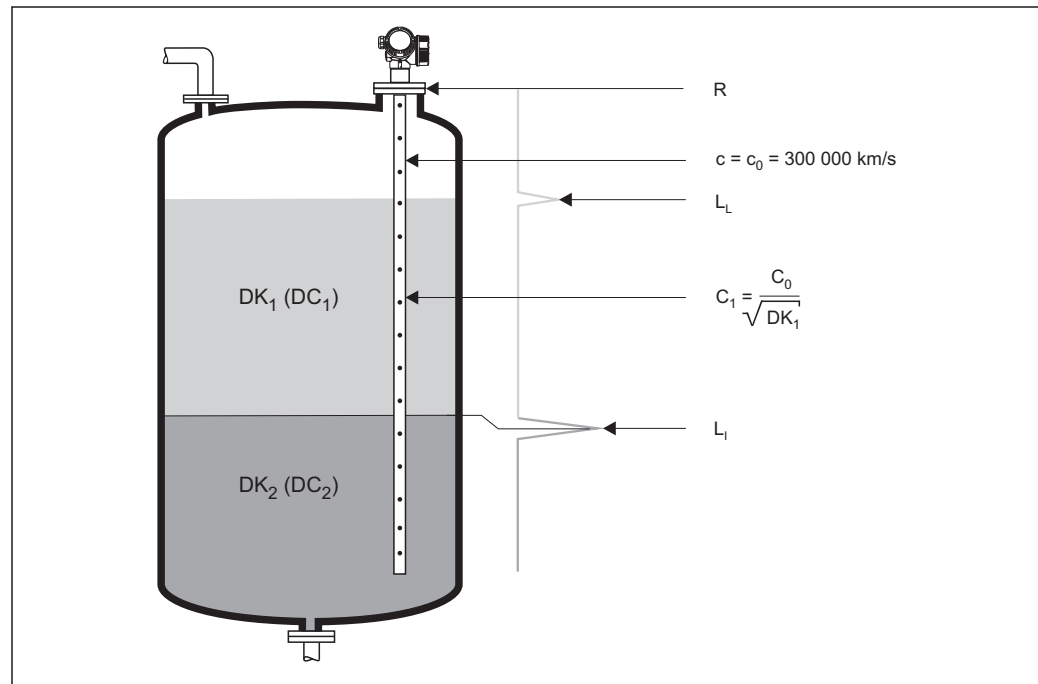
2 Trennschichtmessung mit geführtem Radar
