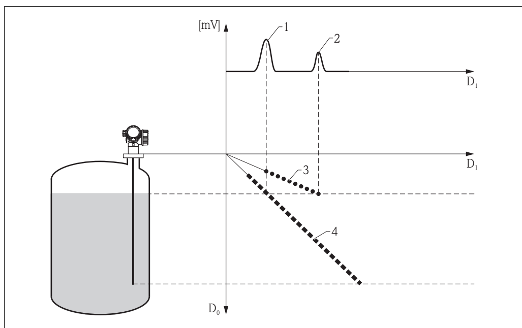
50 Beispiel 2: Tankhistorie mit Mehrfachecho (großer DK-Wert)
