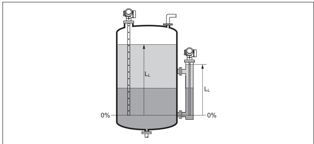
21 Füllstand bei Trennschichtmessungen
