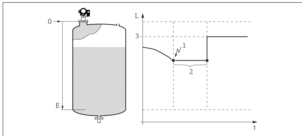
37 "Ausgang bei Echoverlust (→ 118)" = "Wert bei Echoverlust"
