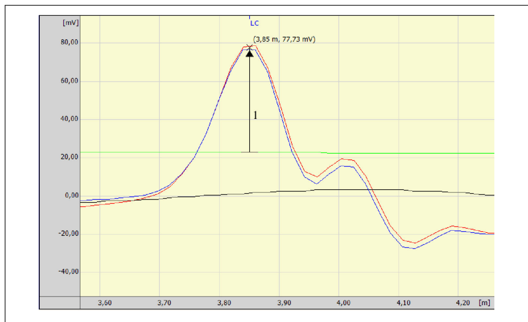
1 Die relative Echoamplitude ist der Abstand von der Echoschwelle (grün) zum Echopeak in der Hüllkurve (rot).
