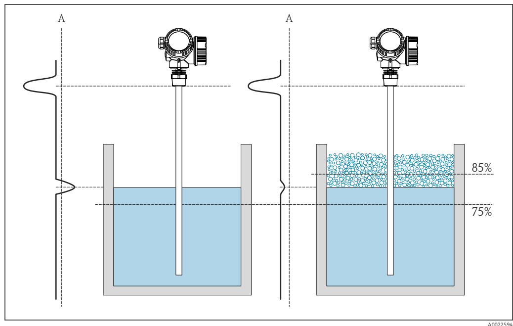
56 Verringerung der Amplitude des Radarsignals bei Schaumbildung
