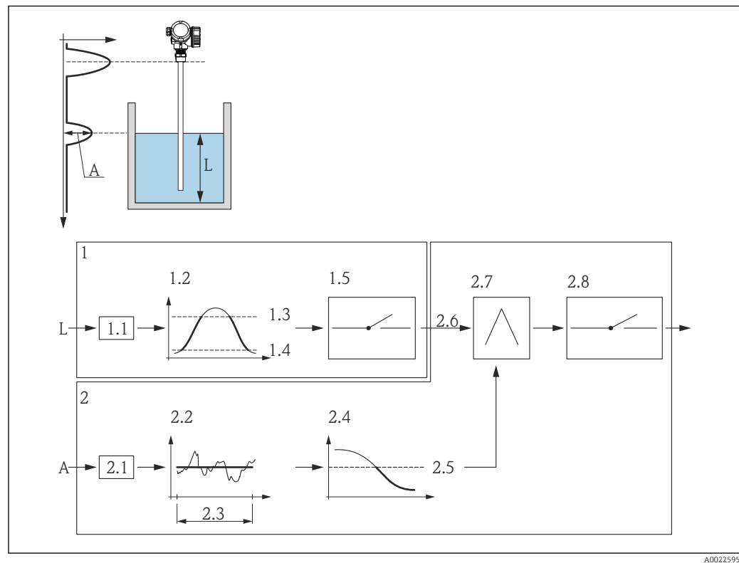
57 Parametrierung der Erweiterten Diagnose zur Schaumerkennung
