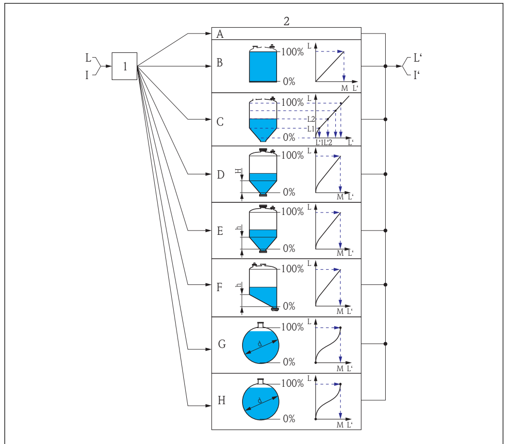
23 Linearisierung: Umrechnung des Füllstands und gegebenenfalls der Trennschicht in ein Volumen oder ein Gewicht; die Umrechnung ist von der Behälterform abhängig
