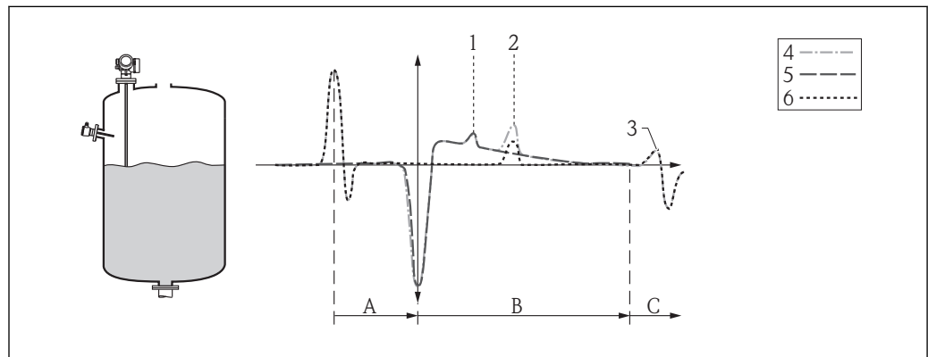
42 Ausblendung und Differenzkurve
