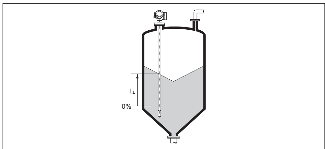
22 Füllstand bei Schüttgutmessungen
