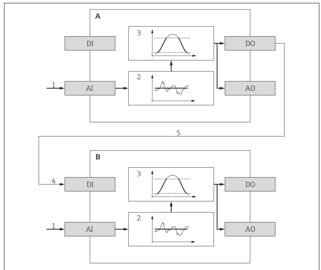
54 Verlinkte Erweiterte-Diagnose-Blöcke
