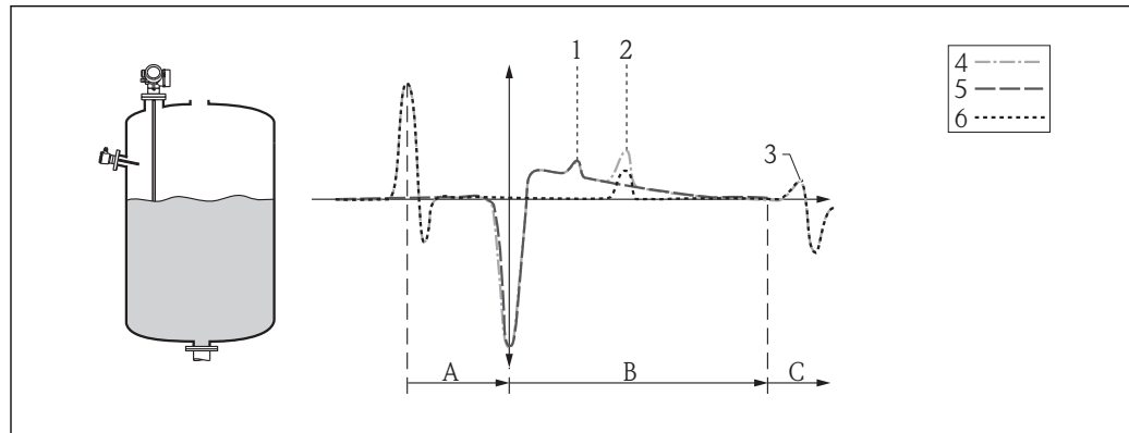
4 Ausblendung und Differenzkurve
