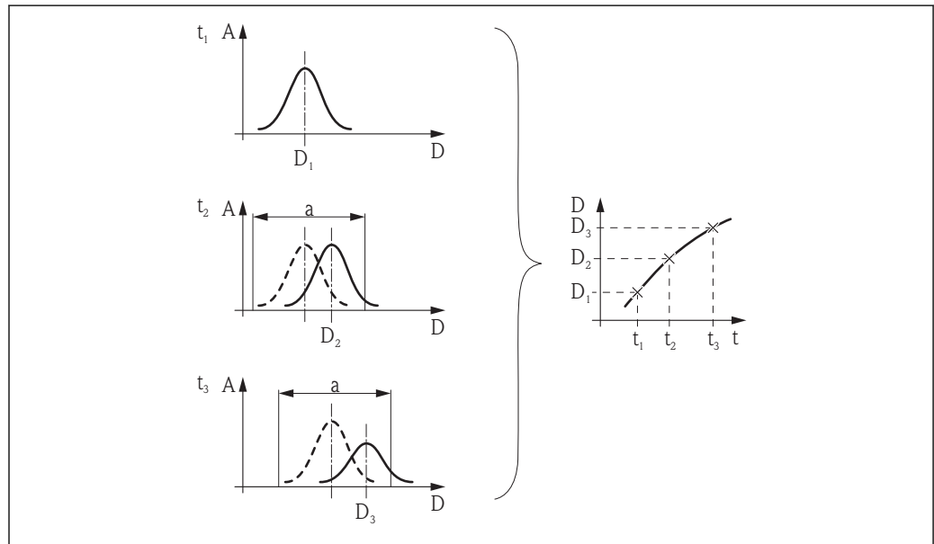
48 Definition eines Track: Das Echo wird in der jeweils nächsten Hüllkurve innerhalb des Fensters der Breite "a" um die vorherige Echoposition gesucht. Der zeitliche Verlauf der Echoposition definiert den Track.
