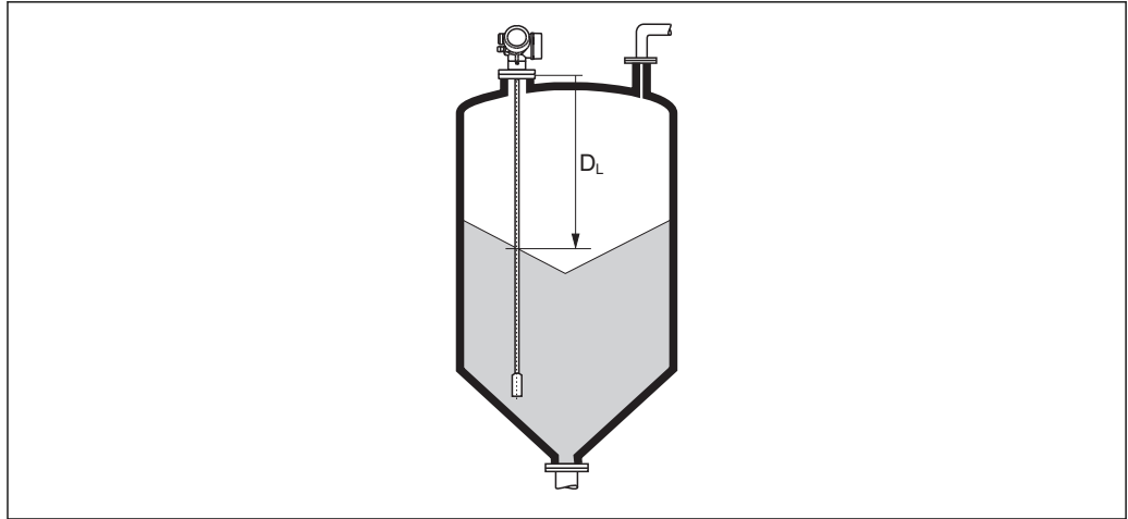
29 Distanz bei Schüttgutmessungen
