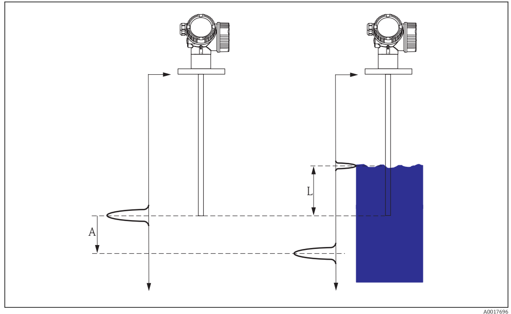
47 Verschiebung des Sondenendsignals (EOP) in Abhängigkeit vom Füllstand
