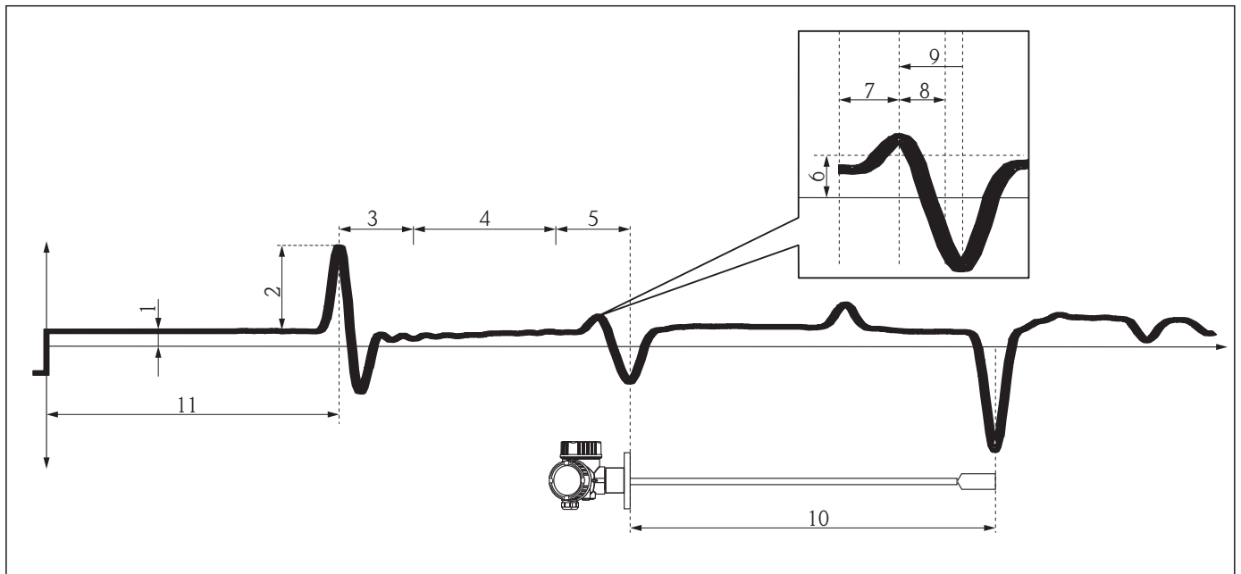
3 Wichtige Merkmale der Hüllkurve
