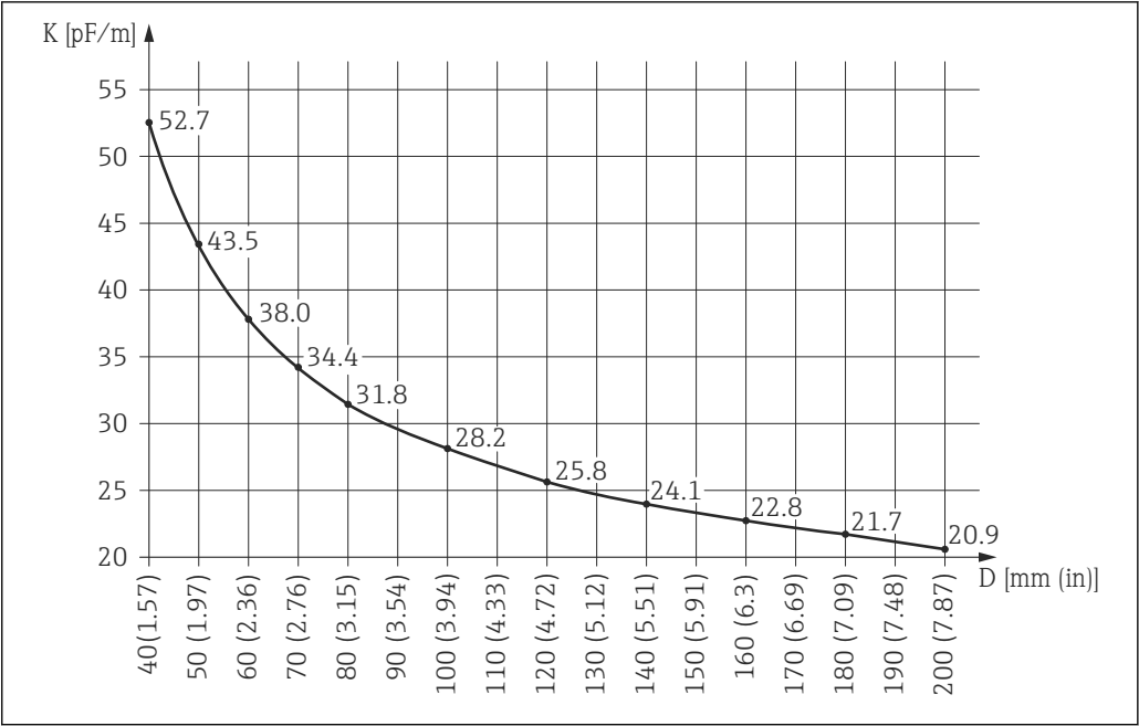
53 Leerkapazität pro Meter in Abhängigkeit von Bypass-/Schwallrohrdurchmesser
