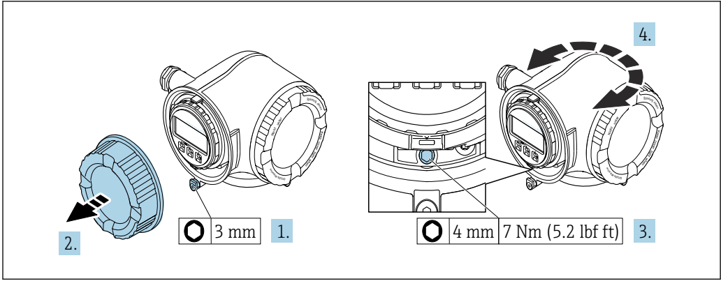
5 非防爆型外壳
