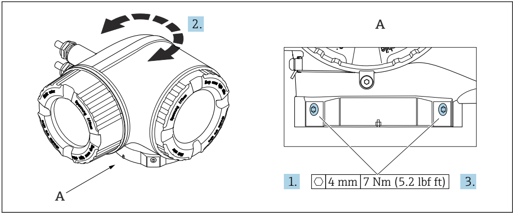
6 防爆型外壳
