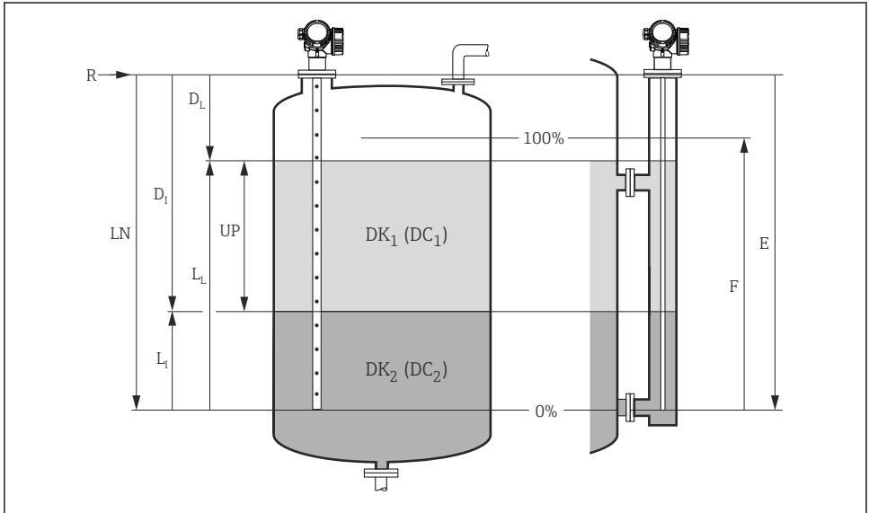
17 Paramètres de configuration pour la mesure d'interface
