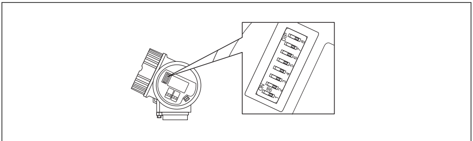
11 Commutateur d'adresses dans le compartiment de raccordement
