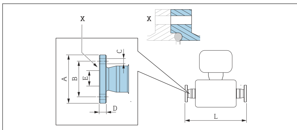
35 Détail X : Raccord process asymétrique, la partie bleue fait partie de la livraison.
