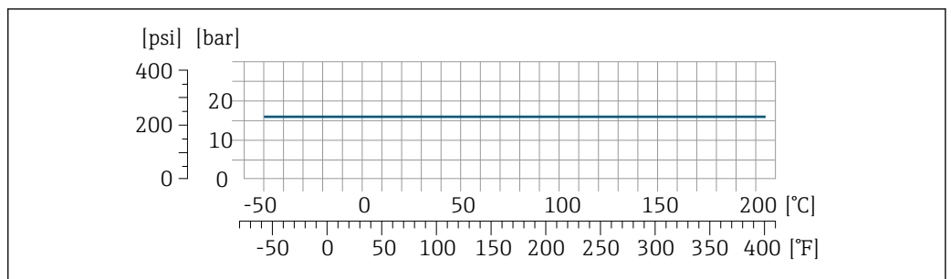
29 Avec matériau de raccord 1.4435 (316L)
