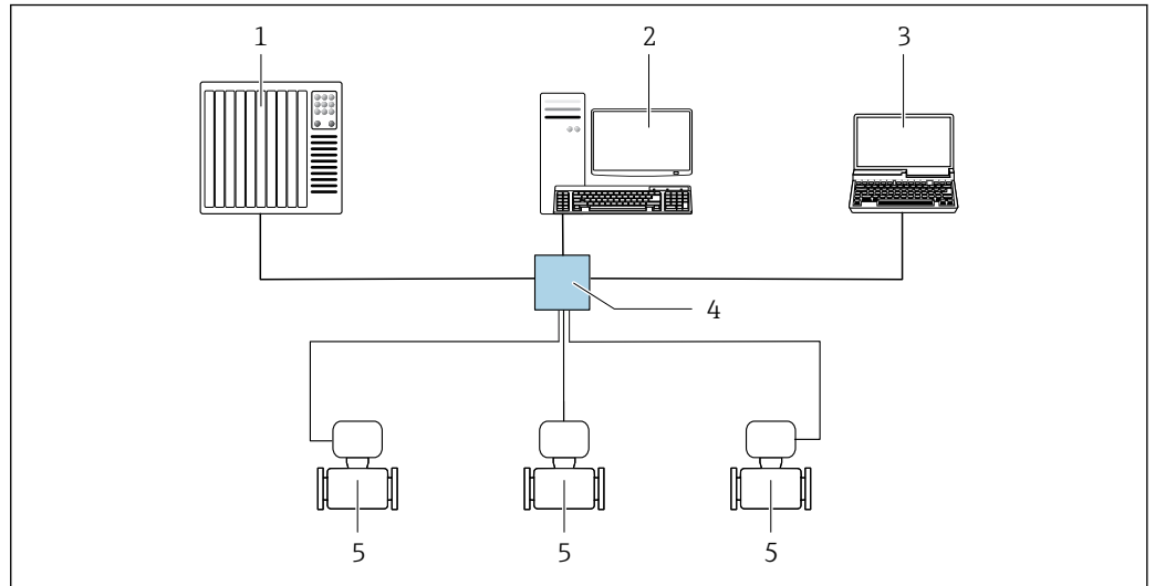
74 Options de configuration à distance via Modbus TCP sur Ethernet - 100 Mbit/s : topologie en étoile
