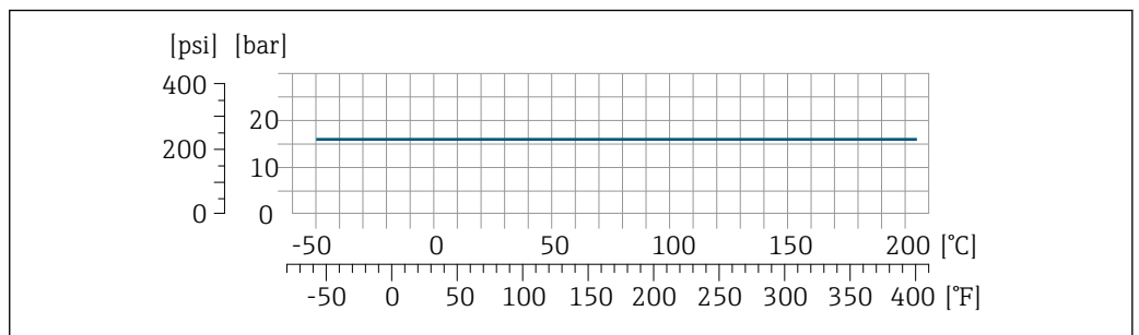
30 Avec matériau de raccord 1.4435 (316L)
