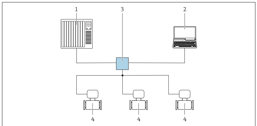
71 Options de configuration à distance via réseau PROFINET : topologie en étoile
