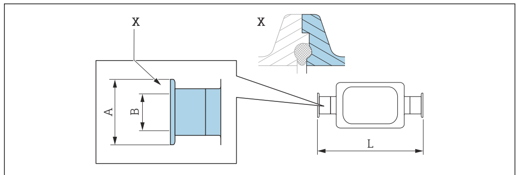
40 Détail X : Raccord process asymétrique, la partie bleue fait partie de la livraison.
