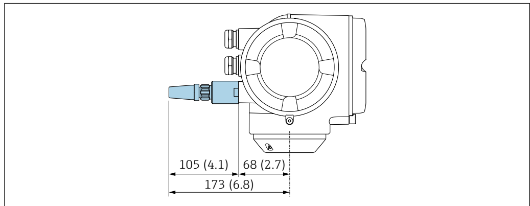
48 Unité mm (in)
