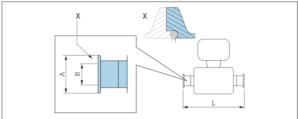
52 Détail X : Raccord process asymétrique, la partie bleue fait partie de la livraison.
