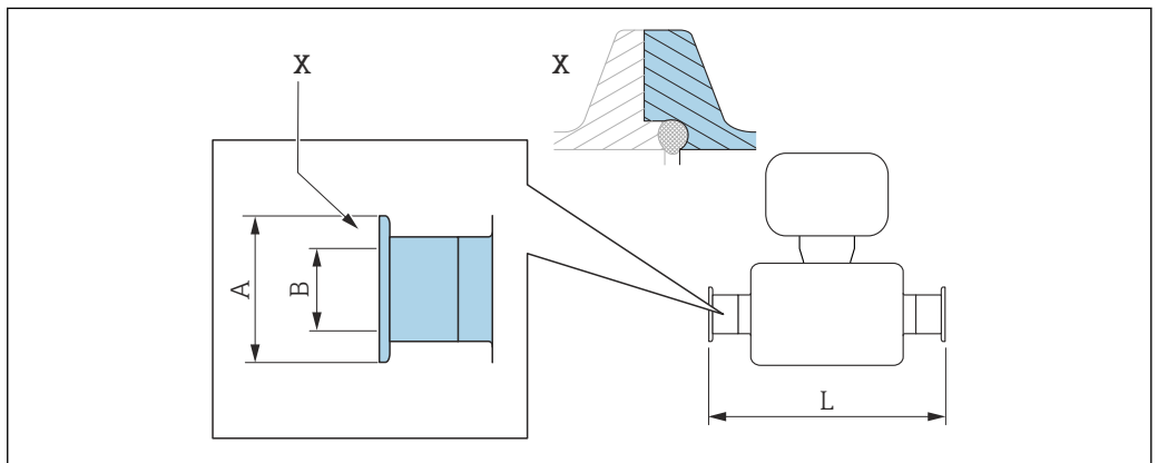
39 Détail X : Raccord process asymétrique, la partie bleue fait partie de la livraison.
