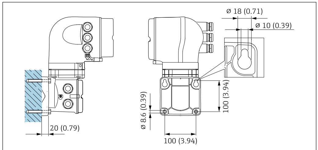
18 Unité mm (in)
