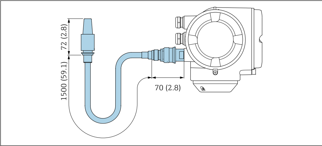
49 Unité mm (in)
