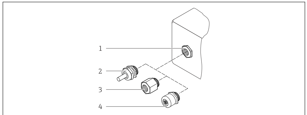
61 Entrées de câble/presse-étoupe possibles
