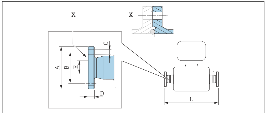
34 Détail X : Raccord process asymétrique, la partie bleue fait partie de la livraison.
