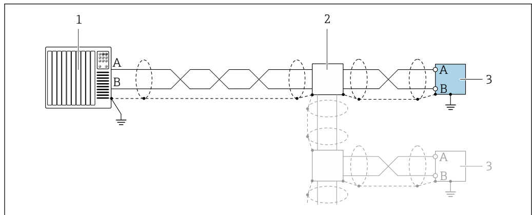
20 Пример подключения для Modbus RS485
