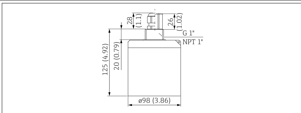
9 Размеры. Единица измерения мм (дюйм)
